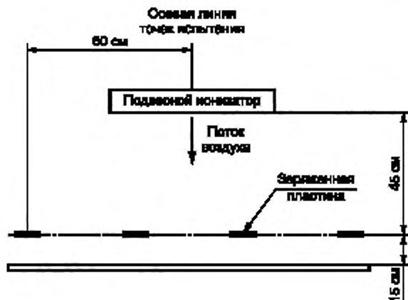
Рисунок 16 — Точки измерений при использовании подвесного ионизатора. Вид сбоку
