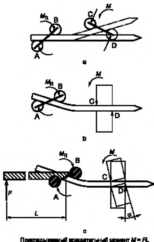
Рисунок 3 — Принцип статического испытания на изгиб методом приложения нагрузки F в четырех точках
