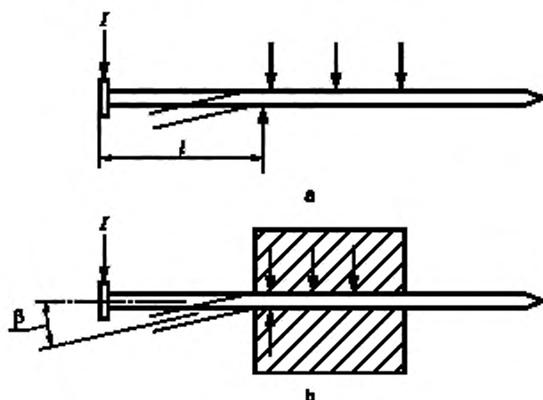
Рисунок 4 — Принцип динамического испытания (трехточечного) на изгиб методом ударной нагрузки F , приводящей к деформации на угол \beta
