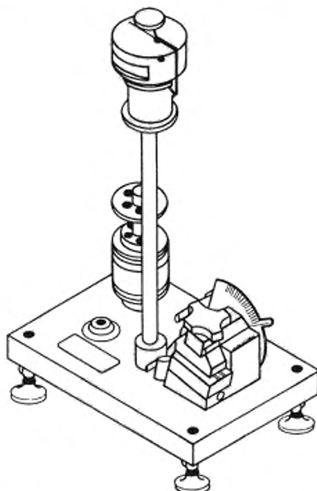
Рисунок 5 — Стандартная испытательная аппаратура. Трехточечное испытание на изгиб методом ударной нагрузки
