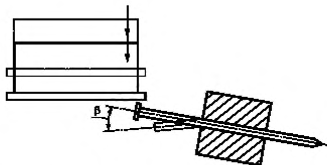
Рисунок 6 — Подробности измерения угла деформации при трехточечном испытании методом ударной нагрузки
