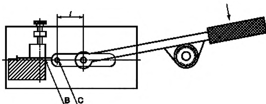
Рисунок 2 — Стандартная испытательная аппаратура. Статическое испытание на изгиб методом приложения нагрузки в трех точках
