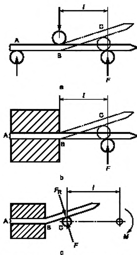
Рисунок 1 — Принцип статического испытания на изгиб методом приложения нагрузки F в трех точках
