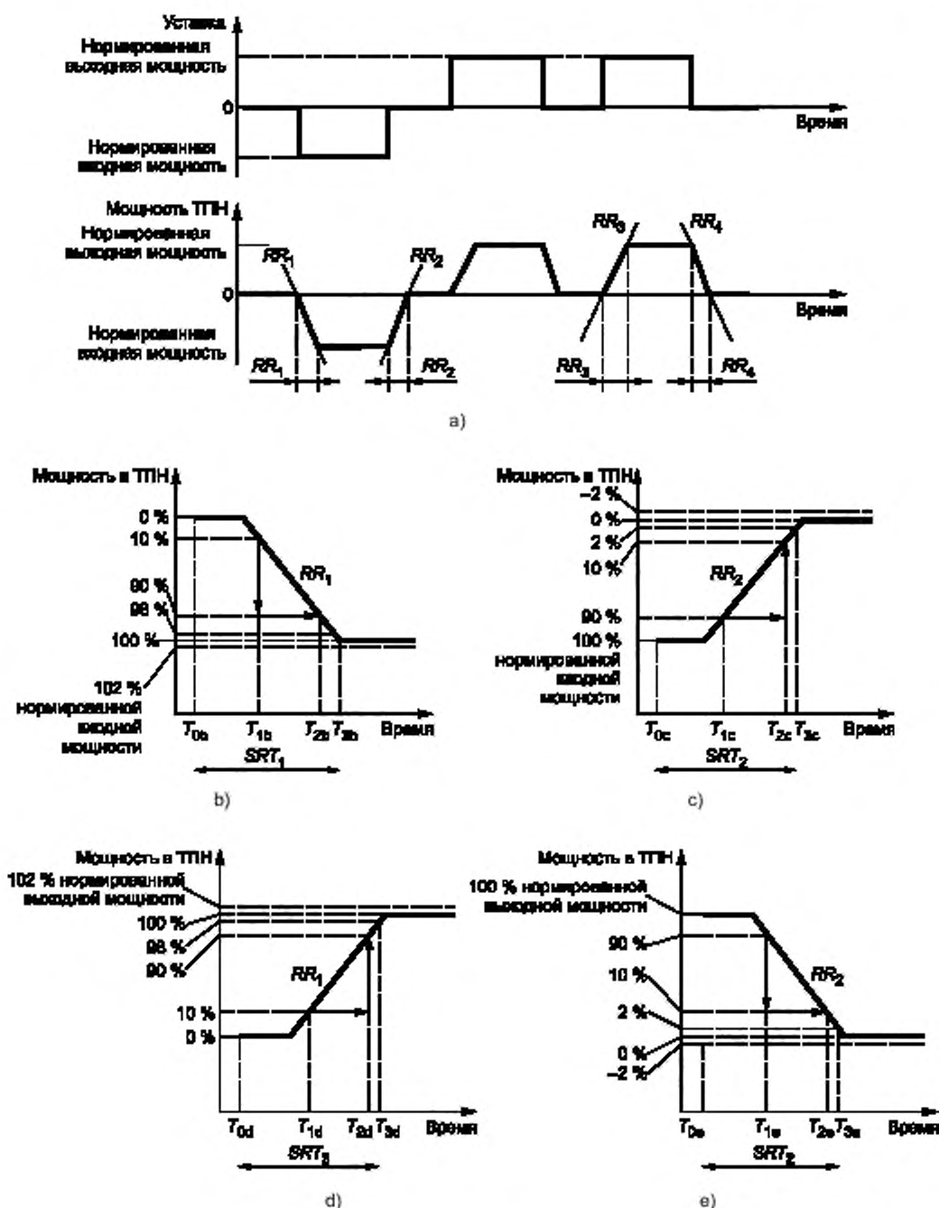
Рисунок 7 — Испытание для определения отклика системы
