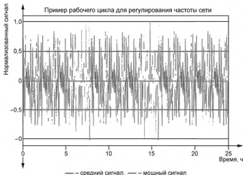
Рисунок А.1 — Рабочий цикл для приложений СНЭЭ класса А
