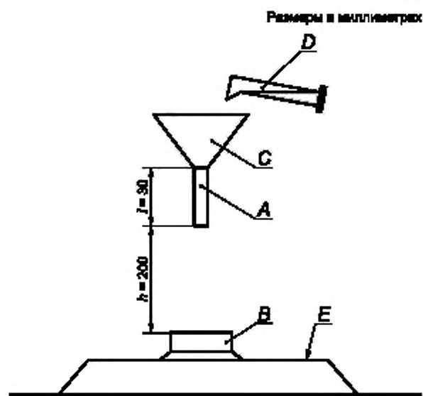
A — воронка с трубкой, внутренний диаметр которой составляет 8 мм; B — испытываемый предмет; C — воронка; D — контейнер с 30 мл соляного раствора; E — горизонтальная поверхность
