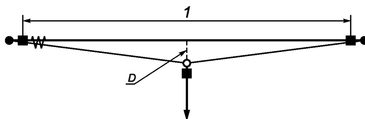
1 — наиболее длинный/короткий пролет; D — динамический прогиб; ■ — датчик нагрузки; —> — направление приложения нагрузки; W — амортизатор энергии (если установлен); ● — концевой анкер; ○ — мобильная анкерная точка
