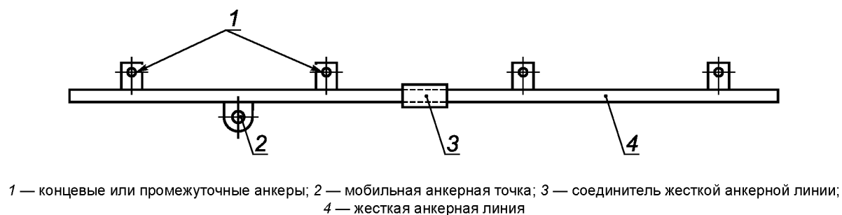
Рисунок 7 — Пример анкерного устройства типа D
