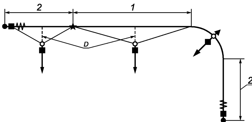
Рисунок 17 — Образец испытательной конфигурации многопролетного анкерного устройства типа С без угла
