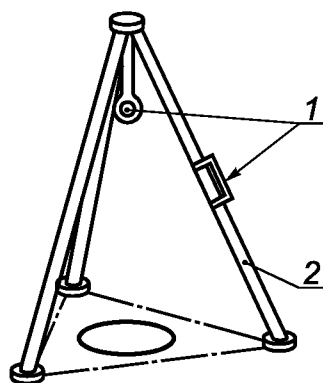
a — трипод
