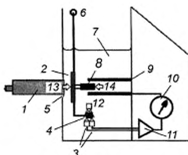
1 — преобразователь; 2 — поглощающая мишень; 3 — фототранзисторы; 4 — затемненный флажок; 5 — тонкое пластиковое окно; 6 — опорная ось; 7 — вода; 8 — магнит; 9 — катушка; 10 — амперметр; 11 — усилитель; 12 — светодиод; 13 — радиационная сила; 14 — магнитная сила
