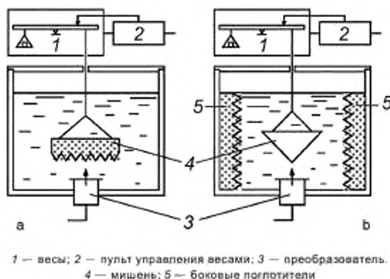
Рисунок F.1 — Компоновка А с поглощающей (а) и отражающей (б) мишенями
