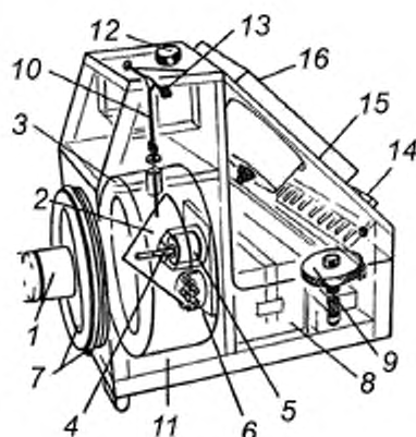
1 — преобразователь; 2 — полая коническая мишень; 3 — поглотитель; 4 — магнит для уравнивания радиационной силы; 5 — катушка для уравнивания радиационной силы; 6 — индикаторы нуля на светодиодах; 7 — мембрана с фланцем; 8 — свинцово-кислотная батарея; 9 — установка нуля; 10 — подвеска мишени; 11 — камера с водой; 12 — крышка с фильтром; 13 — цапфы на камнях; 14 — переключатель диапазонов; электронный блок, показывающее устройство
