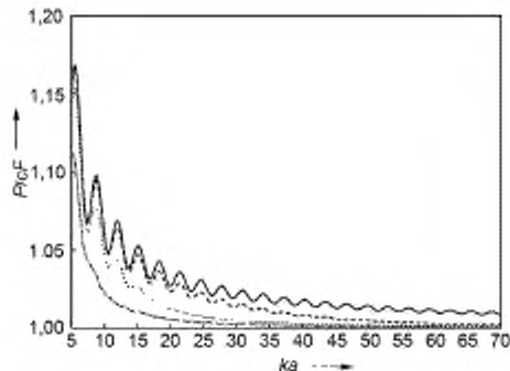
Рисунок Е.2 — Зависимость P/cF от ka для четырех различных псевдотрапециевидных амплитудных распределений: для \epsilon = 0 (поршень) (сплошная кривая), \epsilon = 0,1 (штриховая), \epsilon = 0,25 (точечная), \epsilon = 0,6 (штрихпунктирная)
