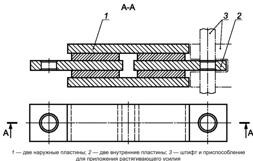
Рисунок 1 — Схема образца
