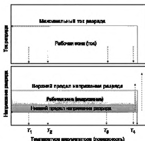
Рисунок A.2 — Примеры параметров рабочей зоны при разряде
