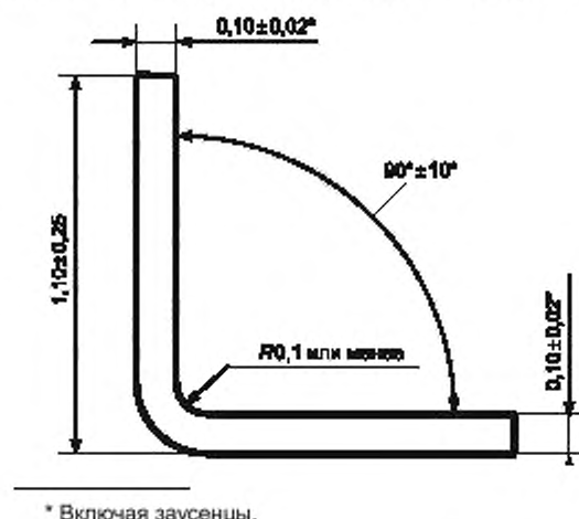
Рисунок A.10 — Размеры готовой никелевой частицы
