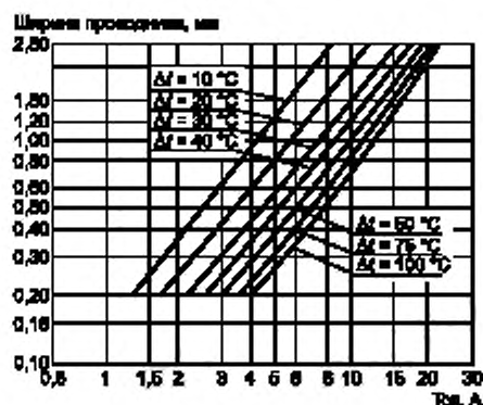
Рисунок 36 г — толщина проводника составляет 105 мкм
