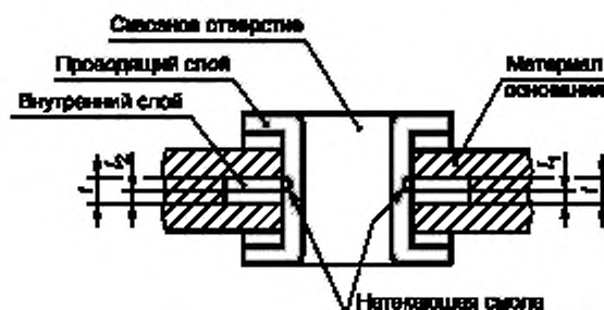
Рисунок 38 а — Вертикальный микрошлиф
