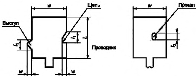
Рисунок 31 а — Щель и выступ
