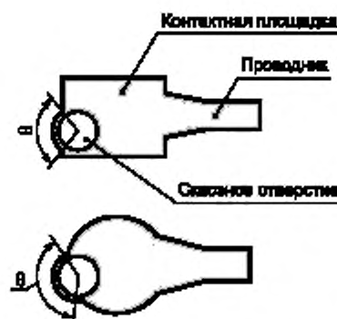
Рисунок 21 с — Допустимая область разрыва пояски
