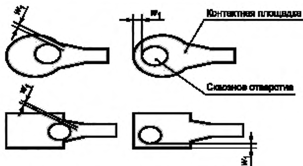
Рисунок 21 а — Минимальный поясок на внешнем слое
