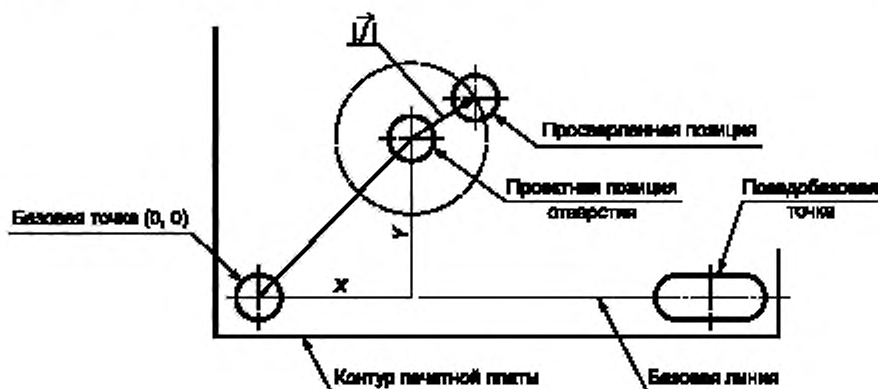
Рисунок 7 — Расположение монтажных отверстий для установки компонентов
