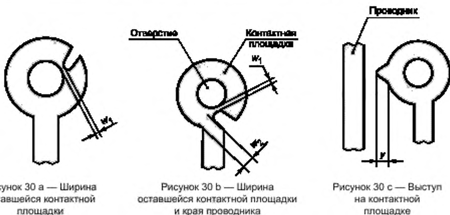
Рисунок 30 — Контактная площадка
