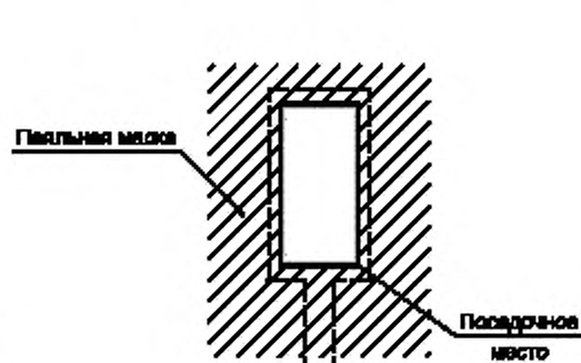
Рисунок 24 б — Смещение и полное покрытие паяльной маской
