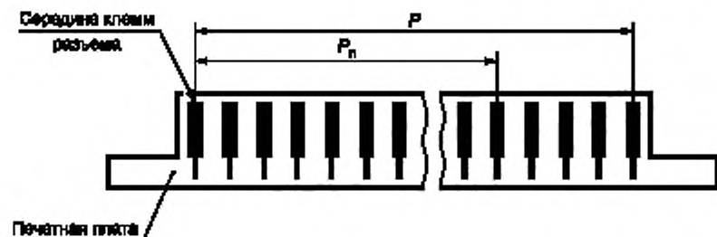
Рисунок 13 — Расстояние между серединами клемм
