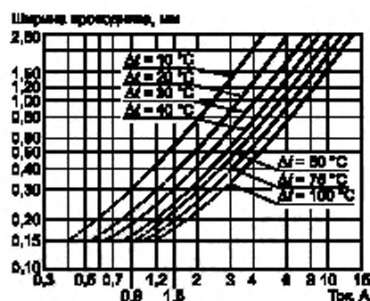
Рисунок 36 б — толщина проводника составляет 35 мкм
