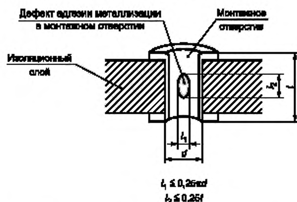
Рисунок 37 — Дефект металлизации монтажного отверстия
