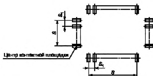
Рисунок 16 — Посадочное место
