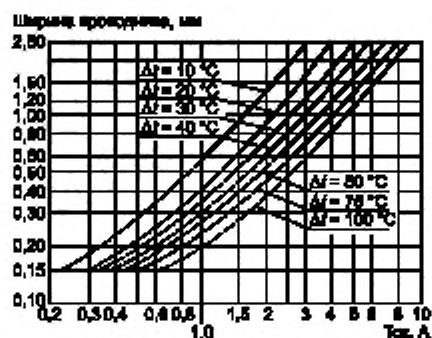
Рисунок 36 а — толщина проводника составляет 18 мкм
