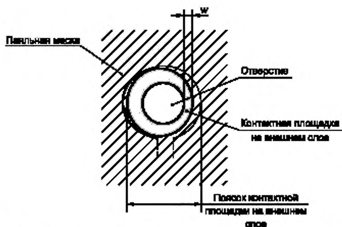
Рисунок 23 — Минимальная контактная площадка, сформированная смещением паяльной маски
