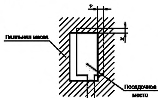
Рисунок 24 а — Смещение паяльной маски
