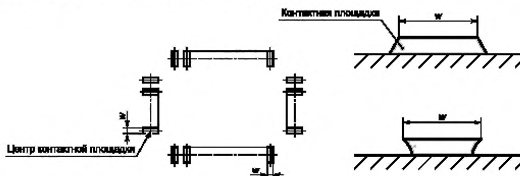
Рисунок 17 — Ширина контактной площадки посадочного места
