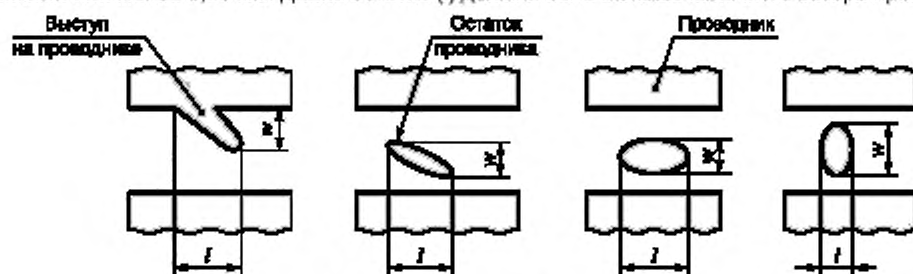
Рисунок 29 — Остаток проводника
