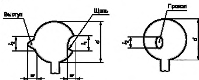
Рисунок 32 а — Щель и выступ
