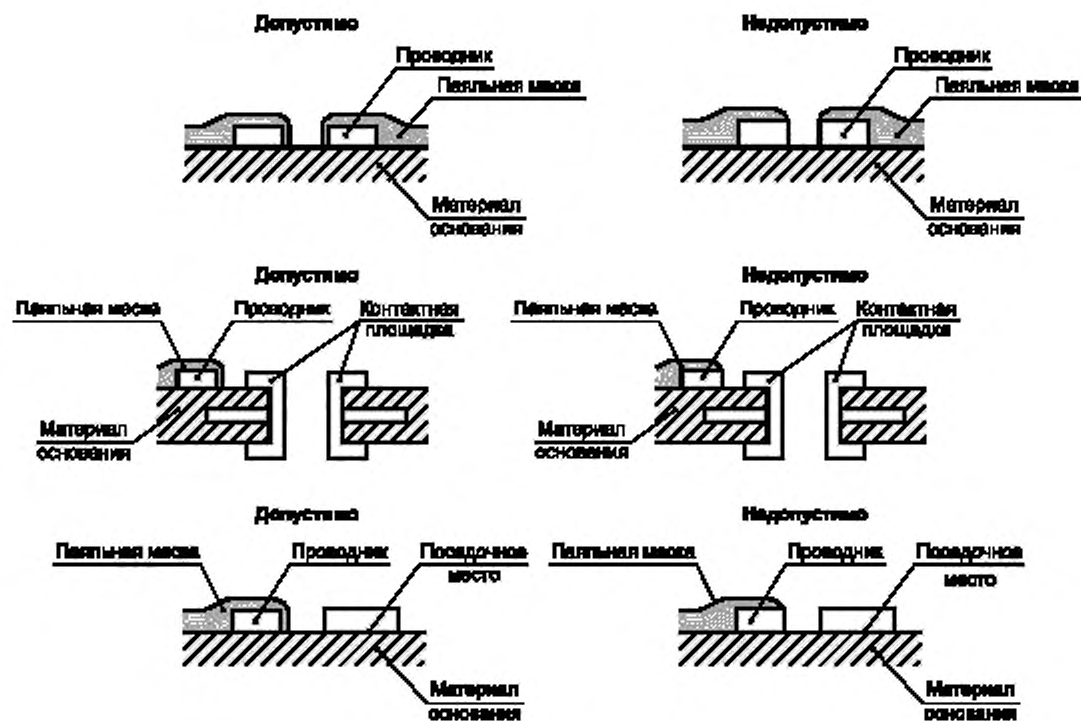
Рисунок 22 — Изображение проводника
