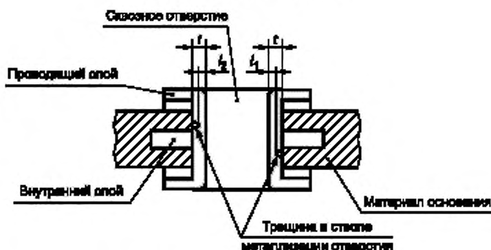
Рисунок 40 — Трещина ствола
