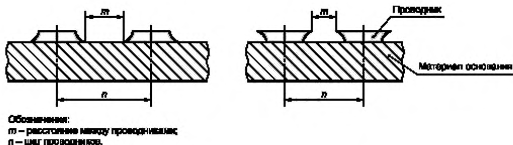
Рисунок 11 — Расстояние между проводником и краем платы
