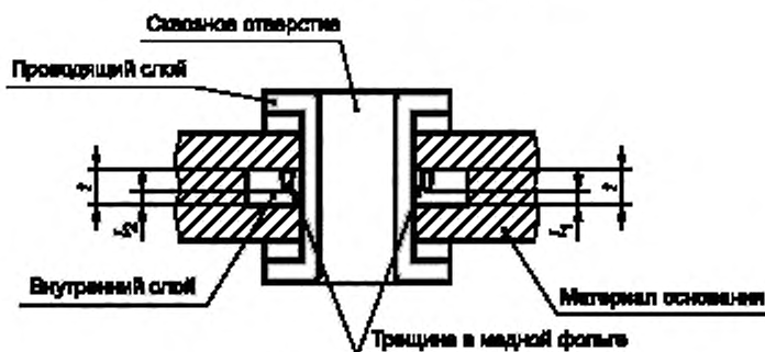
Рисунок 41 — Трещина в медной фольге
