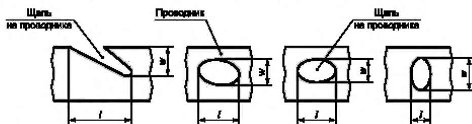
Рисунок 28 — Щели проводников
