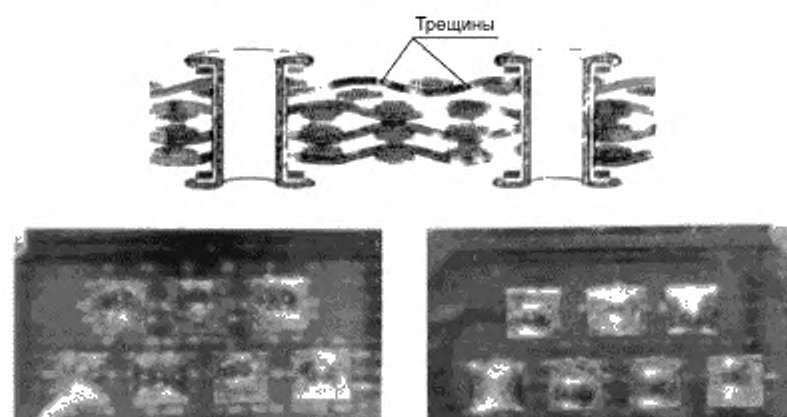
Рисунок 27 — Примеры трещин
