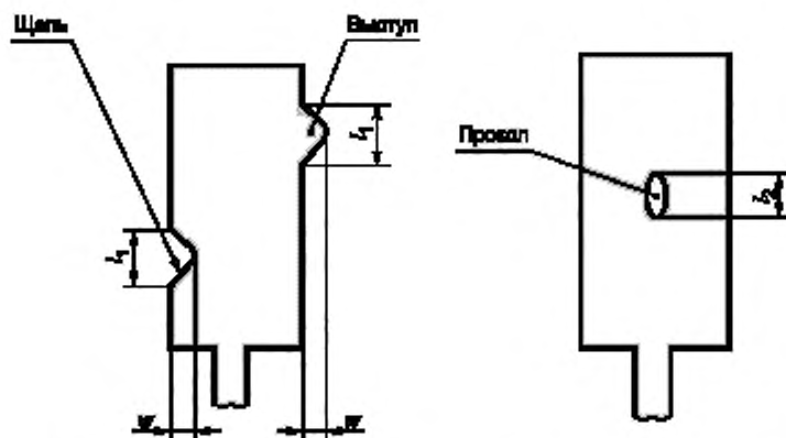
Рисунок 34 а — Щель и выступ
