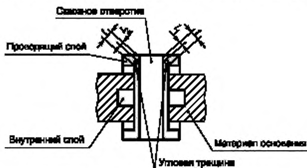
Рисунок 39 — Угловая трещина
