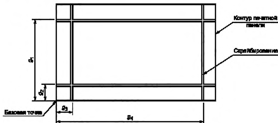
Рисунок 4 — Расстояние от базовой точки до скрайбирования
