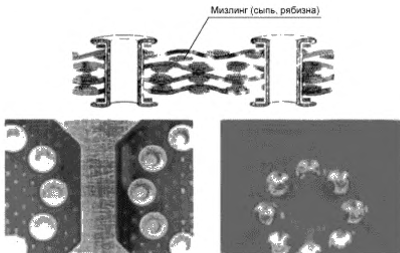
Рисунок 26 — Пример мизлинга
