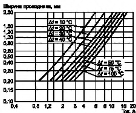
Рисунок 36 в — толщина проводника составляет 70 мкм
