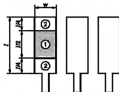
Рисунок 33 — Проверяемые области дефектов печатного контакта
