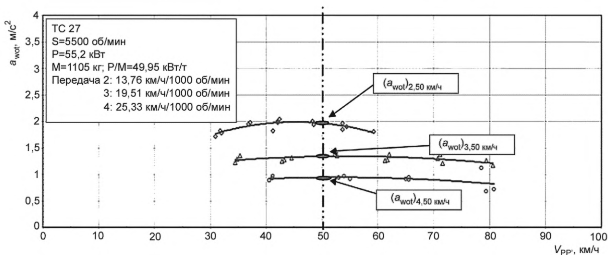
Рисунок А.10 — Ускорение транспортного средства при полностью открытом дросселе a_{wot} = f(v)
