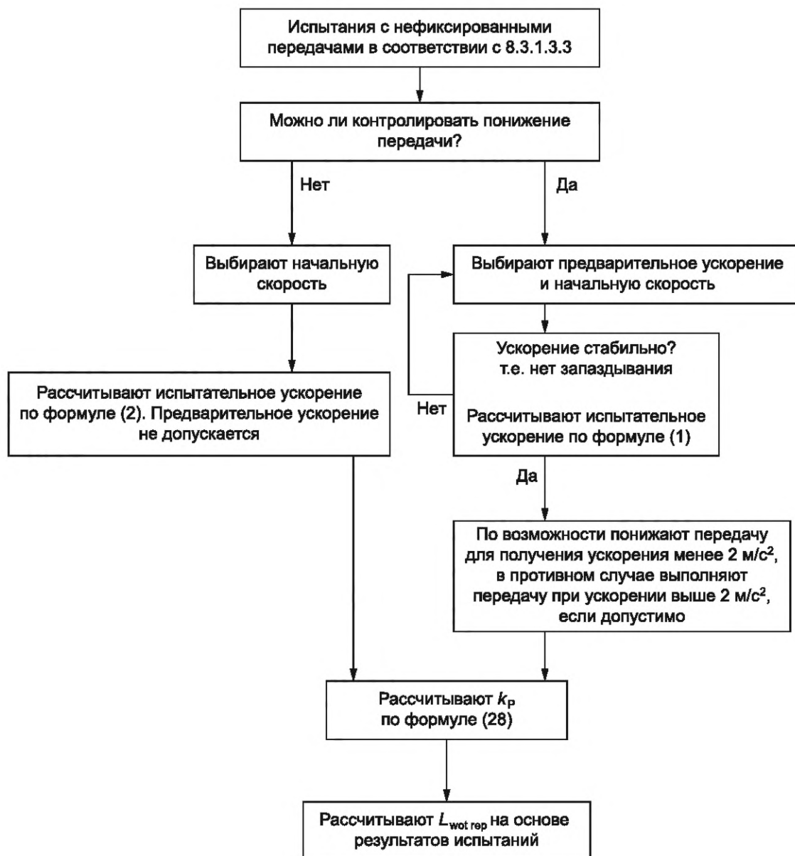
Рисунок С.5 — Алгоритм для определения надлежащего ускорения и L_{wot\ rep} с использованием передач без фиксирования
