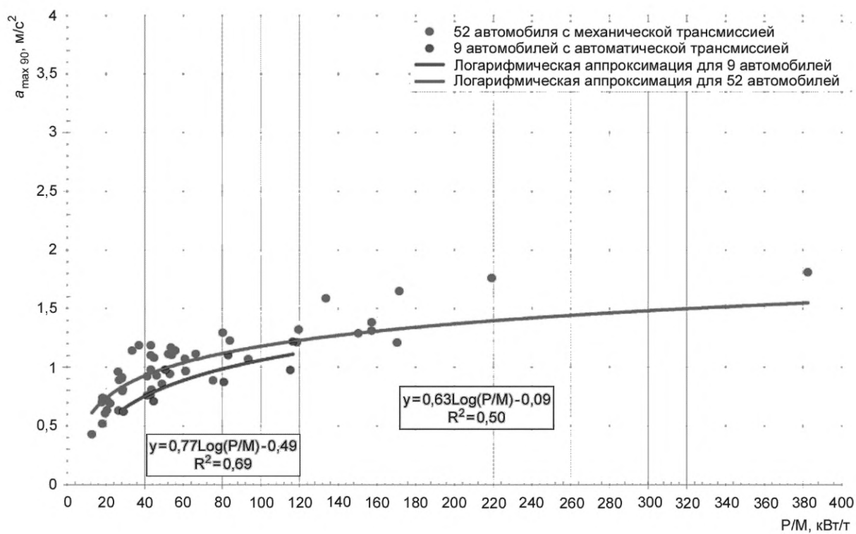
Рисунок А.14 — Регрессионная кривая a_{urban} = f(I_{PMR}) для 52 транспортных средств
