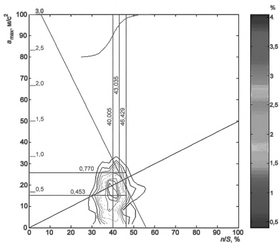
Рисунок А.13 — Определение (n/S)_{L90,a90} при скорости 50 км/ч
