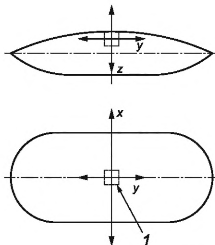
1 — место расположения акселерометра
