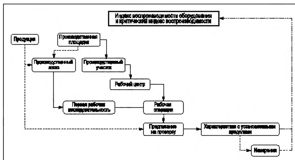
Рисунок А.19 — Диаграмма модели действия элементов КPI-показателя «Индекс воспроизводимости оборудования и критический индекс воспроизводимости оборудования»
