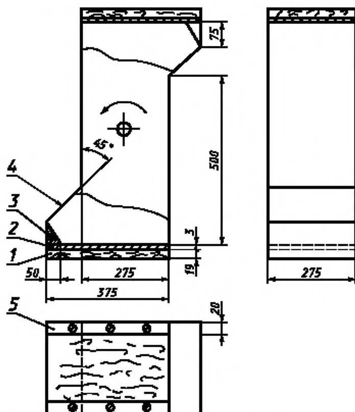
Рисунок 4 — Вращающийся барабан
