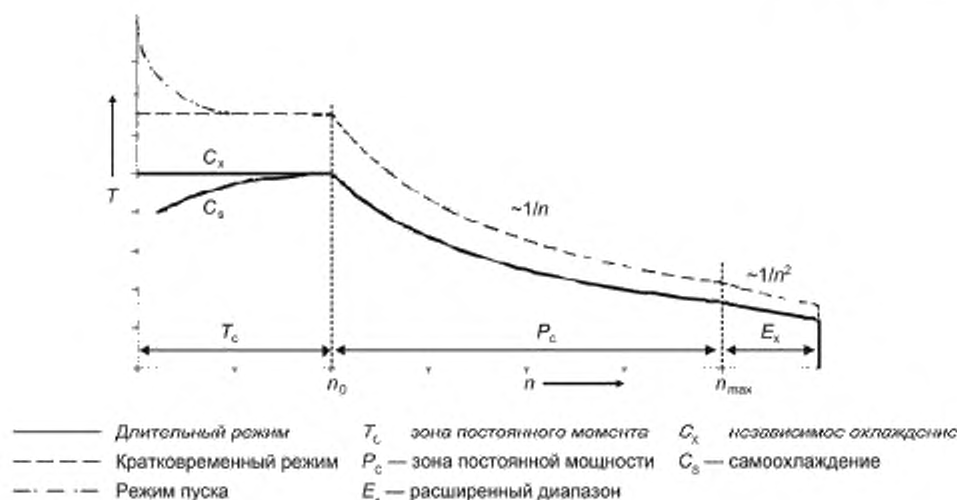
Рисунок 1 — Допустимая область формирования механических характеристик
