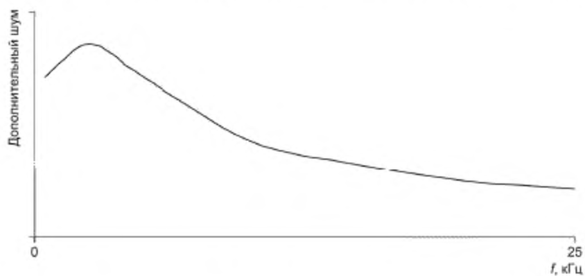
Рисунок A.2 — Влияние частоты коммутации на акустический шум
