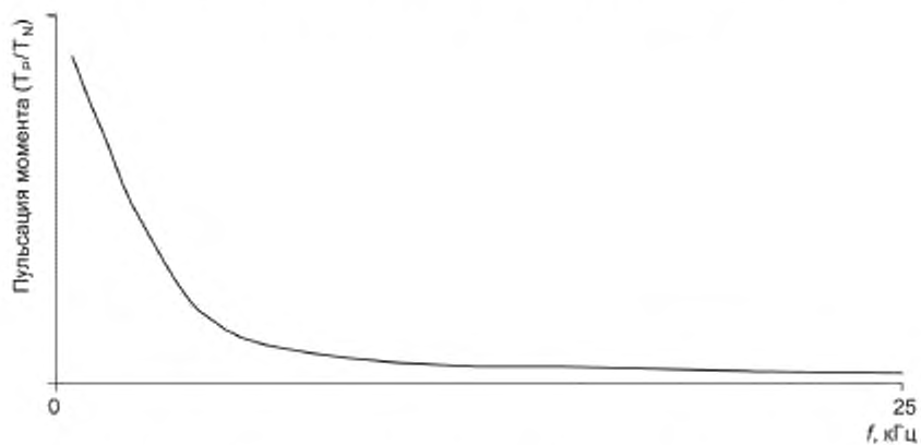
Рисунок A.3 — Влияние частоты коммутации на пульсации крутящего момента
