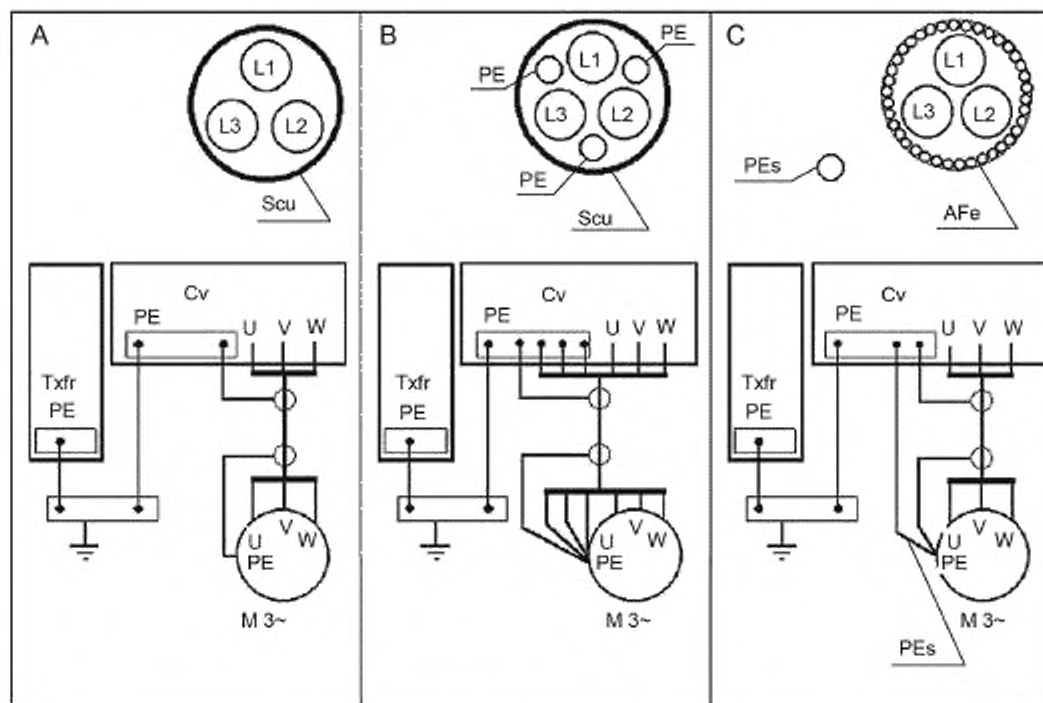
Scu — концентрический медный (или алюминиевый) экран; AFe — стальная броня; Txfr — трансформатор; Cv — преобразователь; PEs — отдельный заземляющий провод
