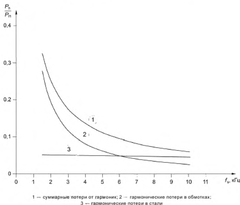
Рисунок 4 — Пример зависимости потерь в электрической машине, вызванных гармониками P_h относительно потерь P_n , на рабочей частоте f_1 и частоте коммутации f_s в случае питания от двухуровневого инвертора напряжения
