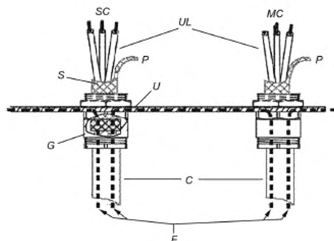
SC — питающий кабель; MC — кабель двигателя; UL — не экранированная часть (по возможности короткая); S — экран кабеля; P — гибкий проводник (по возможности короткий); U — панель сальников; G — ЭМС-сальник кабеля; C — кабели (внешняя оболочка); F — сплошная клетка Фарадея
