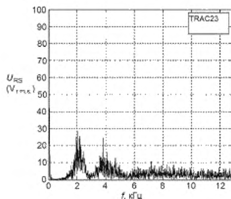
a — Случайная ШИМ
