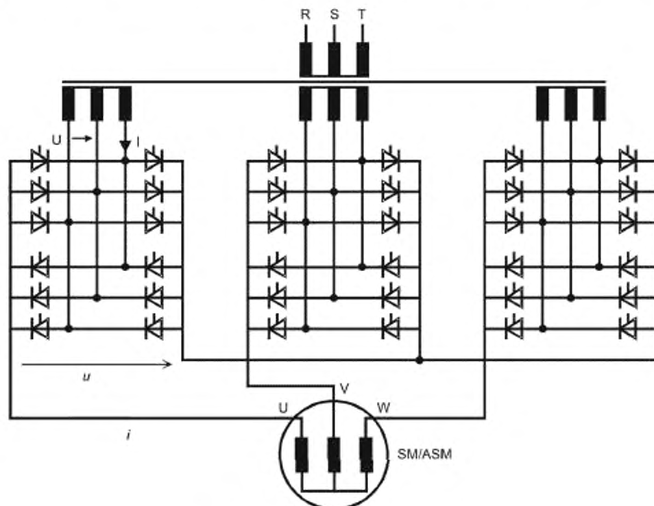
Рисунок 36 — Схема циклоконвертора
