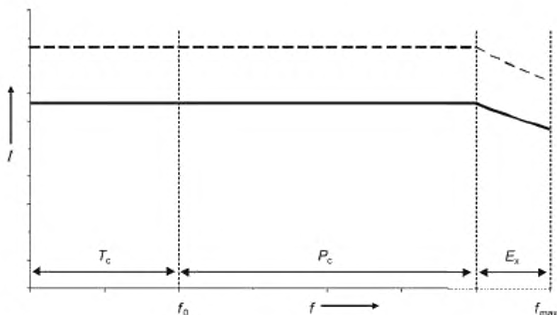
Рисунок 2 — Допустимый выходной ток преобразователя
