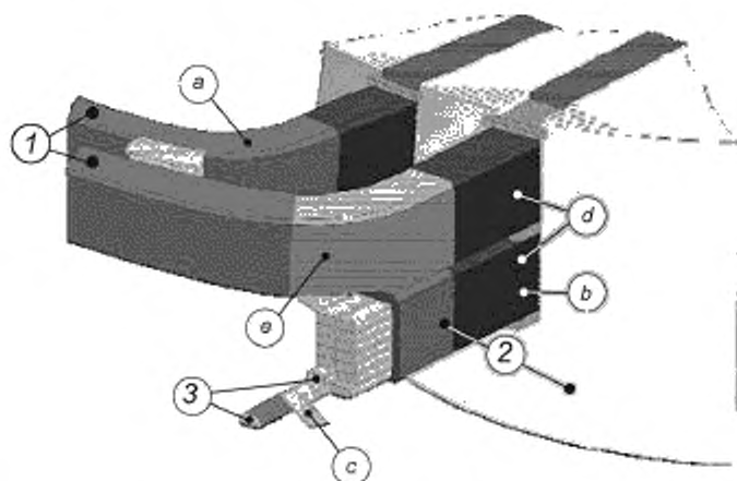
1 — межфазная изоляция; 2 — изоляция фазы относительно земли; 3 — межвитковая изоляция; a — фазная изоляция/изоляция конца обмотки; b — изоляция на землю; c — витковая изоляция; d — слой, содержащий пазовое перенапряжение, e — слой, контролирующий перенапряжение на конце обмотки (выравнивание перенапряжений)
