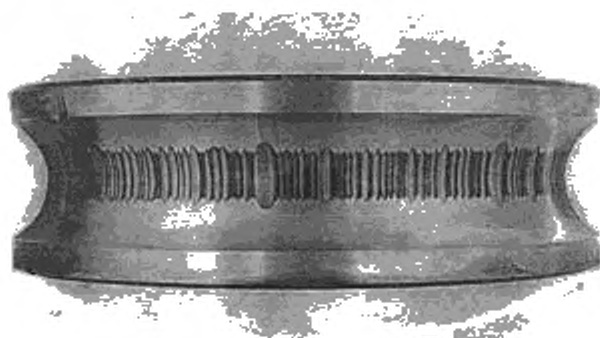
Рисунок 18 — Появление бороздок из-за чрезмерного тока в подшипниках
