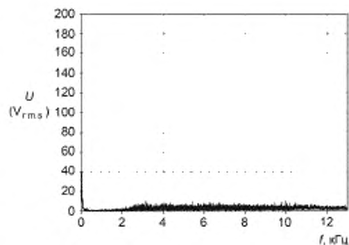
b — Релейное управление, прямое управление моментом, 2,7 кГц в среднем
