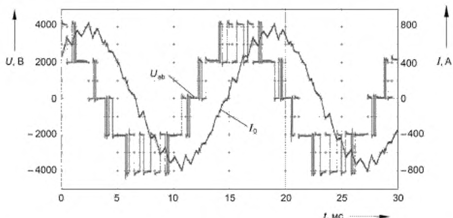
Рисунок 27 — Графики выходного напряжения и тока типичного трехуровневого инвертора напряжения
