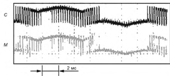
C — фазное напряжение преобразователя, M — фазное напряжение двигателя
