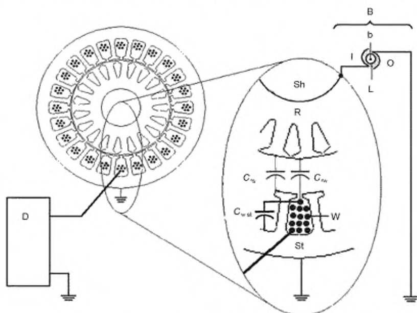
D — преобразователь, Sh — вал; R — ротор; St — статор; W — обмотка; C_{sh} — емкость ротор-статор; C_{rw} — емкость обмотки ротора; C_{wst} — емкость обмотки статора; B — подшипник; b — шарик или ролик; I — внутреннее кольцо, O — внешнее кольцо; L — пленка смазки
