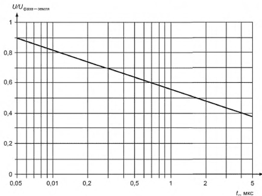
U/U_{\text{фаз-земля}} — напряжение на первичном витке (в процентах от напряжения между фазой и землей); t_r — время нарастания импульса
