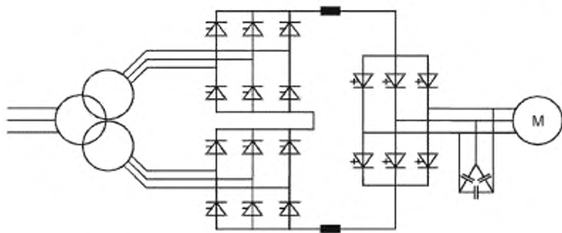
Рисунок 34 — Схема преобразователя с ШИМ-инвертором тока
