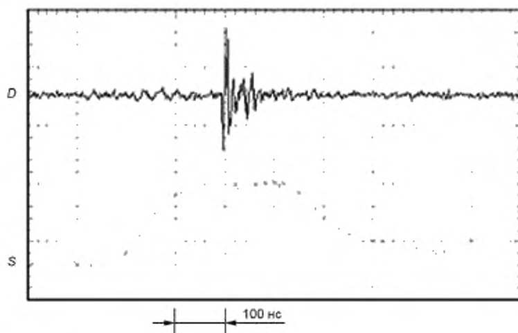
S — импульс напряжения на клеммах двигателя; D — импульс разряда
