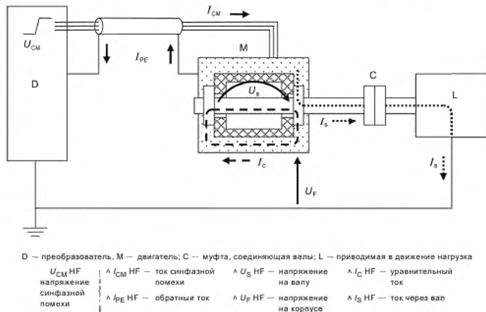
Рисунок 15 — Возможные токи, протекающие через подшипники
