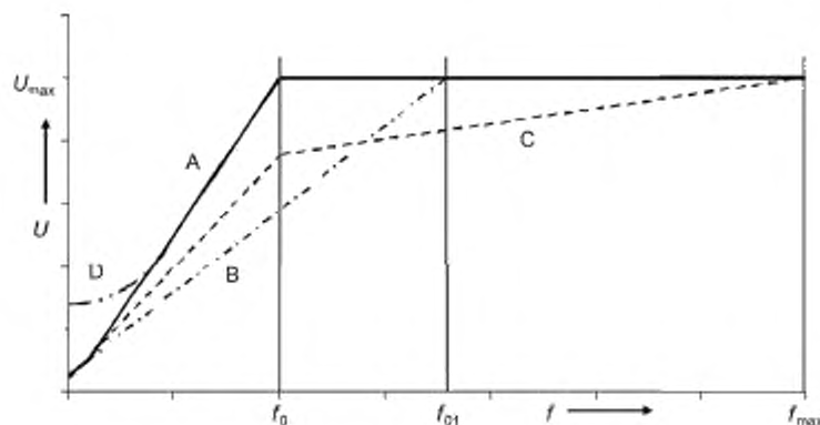
Рисунок 3 — Характеристики «выходное напряжение преобразователя — частота»
