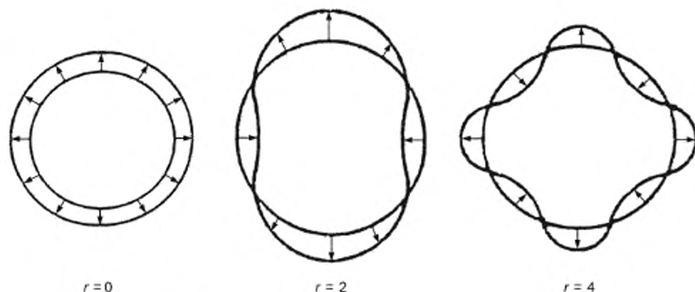
Рисунок 8 — Режимы вибрации сердечника статора
