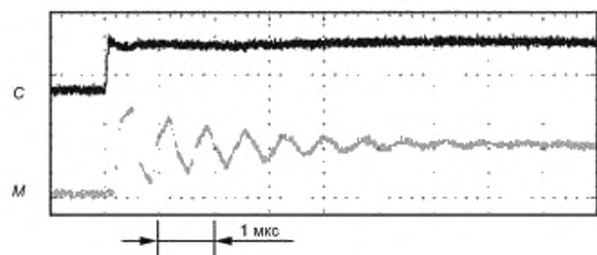
C — фазное напряжение преобразователя; M — фазное напряжение двигателя
