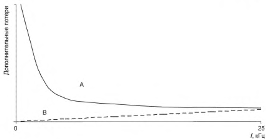
Рисунок A.1 — Влияние частоты коммутации на потери в двигателе и преобразователе
