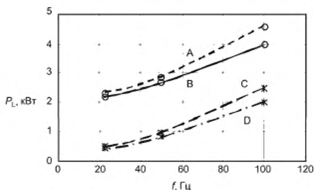
А — полная нагрузка, ШИМ-питание; В — полная нагрузка, синусоидальное питание; С — без нагрузки, ШИМ-питание; D — без нагрузки, синусоидальное питание
