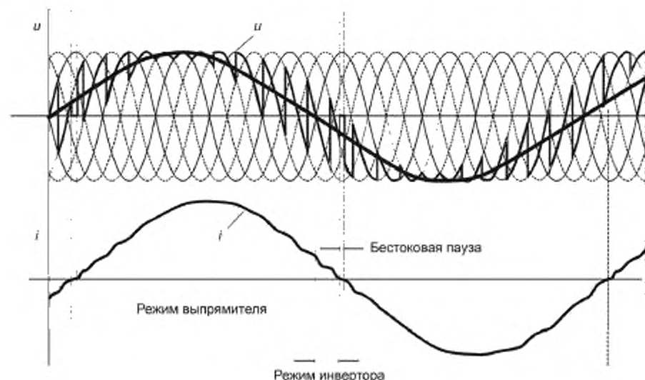
Рисунок 37 — Формы напряжения и тока циклоконвертора
