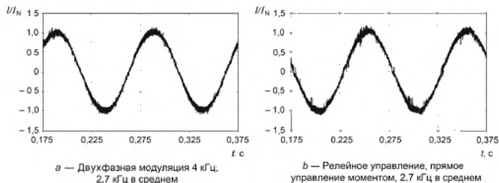
Рисунок В.6 — Типичные осциллограммы тока машины
