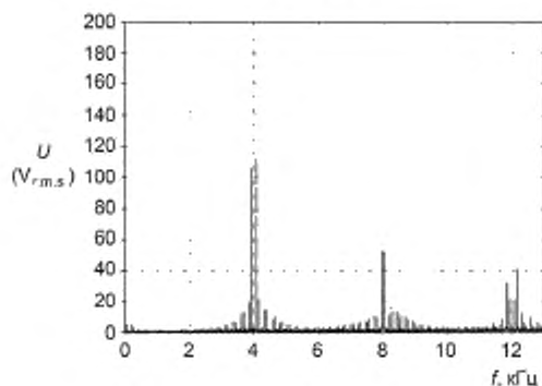
a — Двухфазная модуляция 4 кГц; 2,7 кГц в среднем
