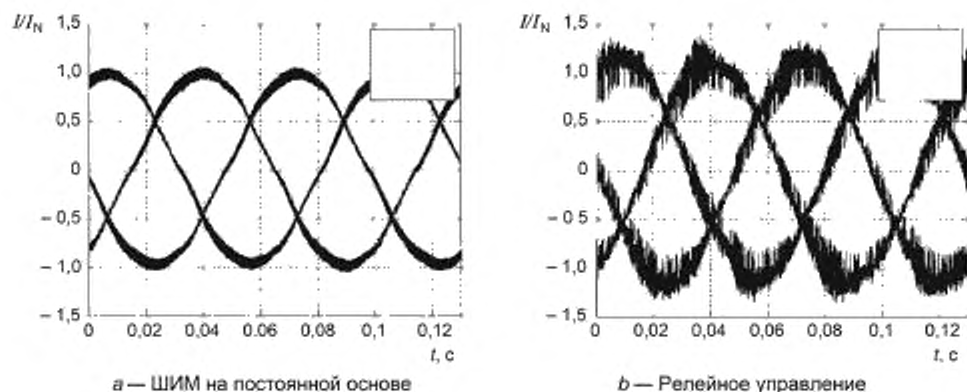
Рисунок В.5 — Типичные осциллограммы тока машины
