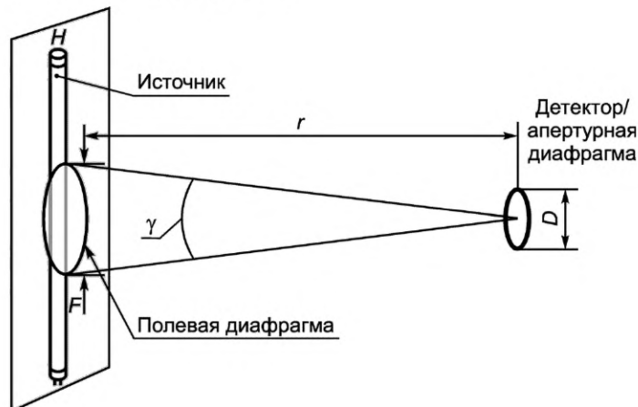
Рисунок 5.3 — Альтернативный метод измерения энергетической яркости
