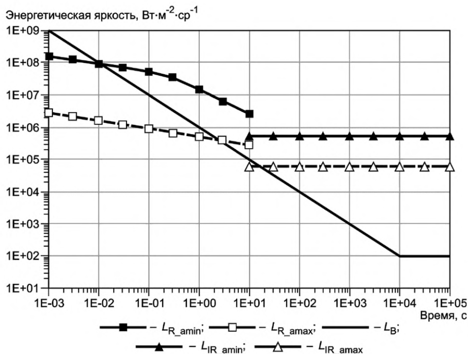
Рисунок 5.5 — Пределы взвешенных значений энергетической яркости в зависимости от времени постоянного воздействия
