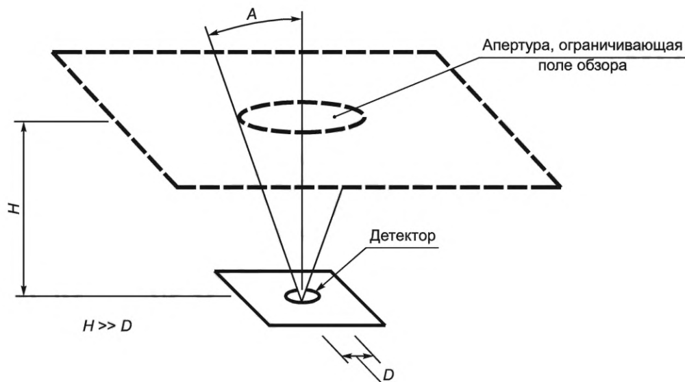
Рисунок 5.1 — Схема измерения энергетической освещенности
