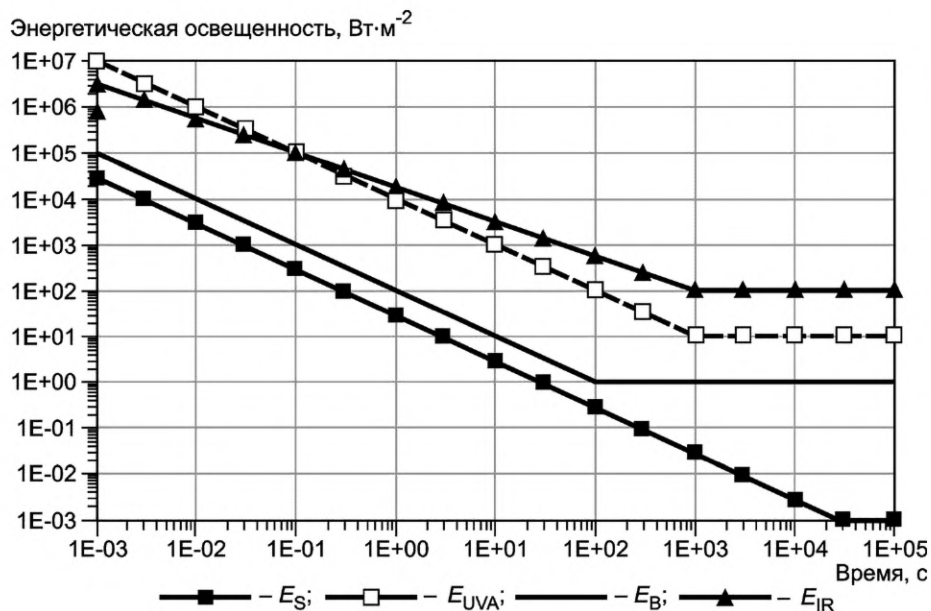
Рисунок 5.4 — Пределы взвешенных значений энергетической освещенности в зависимости от времени постоянного воздействия
