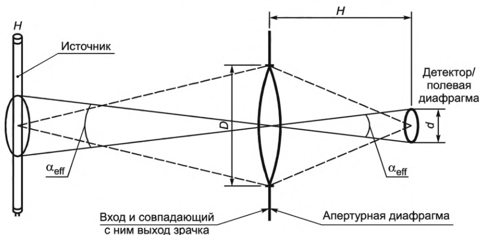
Рисунок 5.2 — Пример формирователя изображения для измерений энергетической яркости
