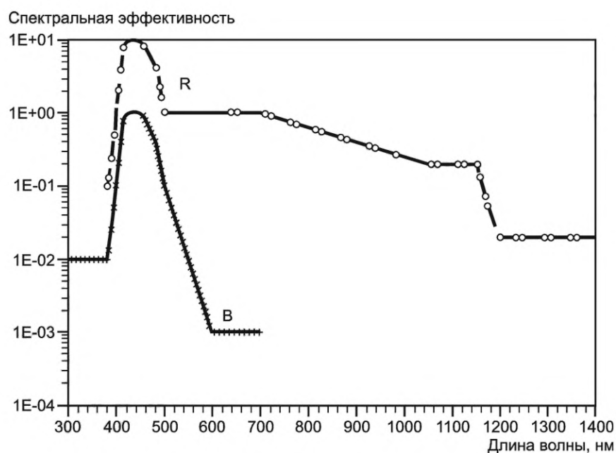
Рисунок 4.2 — Спектральные весовые функции опасности для сетчатки B(\lambda) и R(\lambda)
