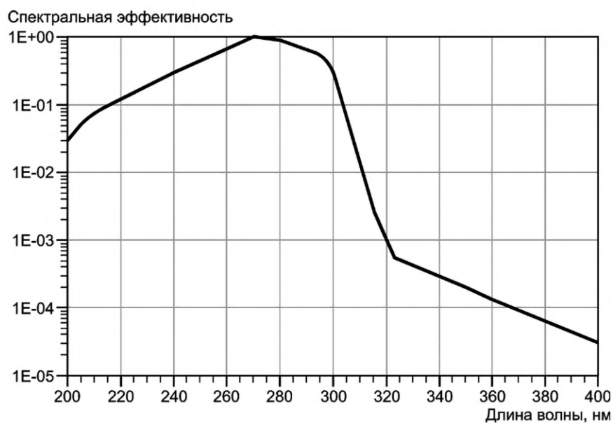
Рисунок 4.1 — Спектральная весовая функция актиничной ультрафиолетовой опасности S_{UV}(\lambda)
