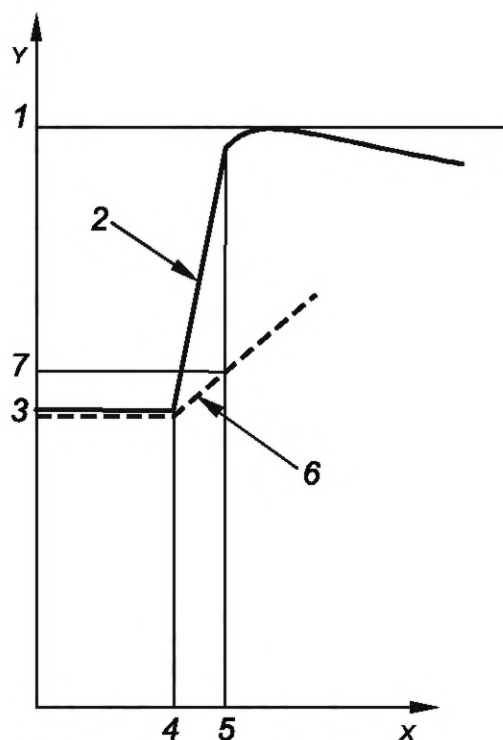
Рисунок 2 — Пример тепловой перегрузки с медленным изменением в случае слишком интенсивного повторно-кратковременного режима работы с запуском (режим работы S4) и прямой тепловой защитой
