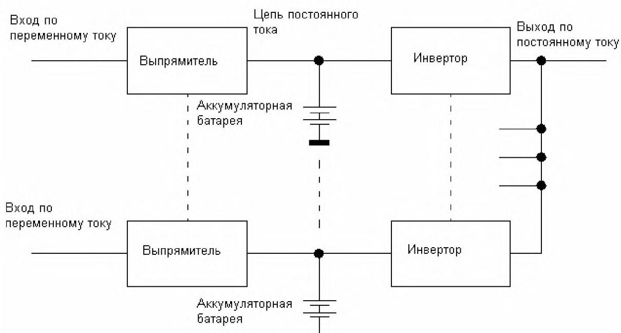
Рисунок А.5а – Частично параллельный АБП (с параллельным инвертором)
