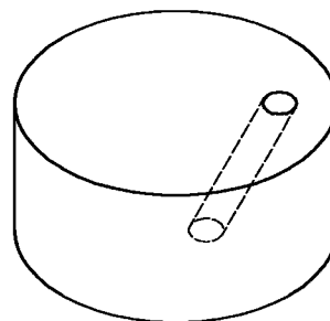
Рисунок А.19 – Отбор пробы из сыра, имеющего форму широкого цилиндра, с помощью пробоотборника вводимого сверху под наклоном
