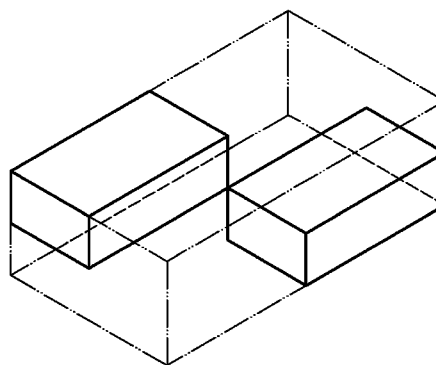
Рисунок А.13 – Отбор пробы из сыра, который имеет форму блока или бруска и у которого большая сторона имеет форму прямоугольника, но не квадрата, путем вырезания куска
