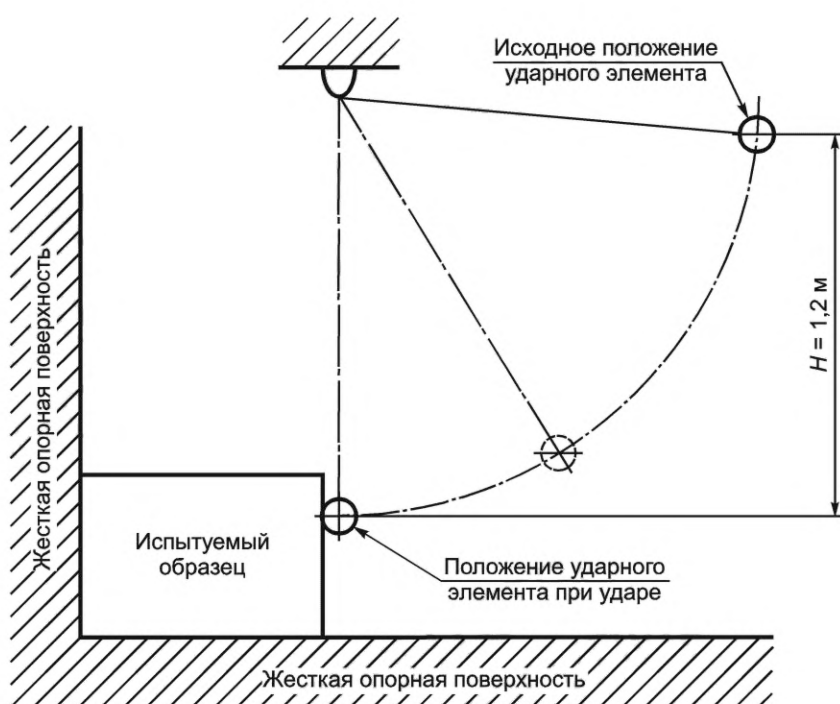
Рисунок 102 — Испытание на удар вертикальной поверхности
