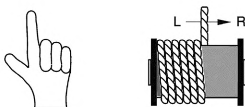
Рисунок В.1b — Канат левой свивки — подмотка
