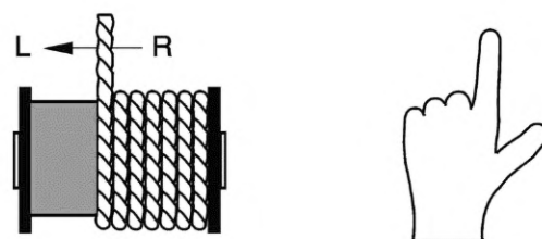
Рисунок В.1d — Канат левой свивки — перемотка
