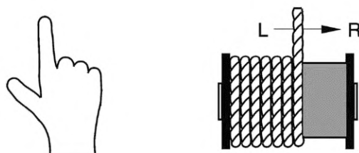
Рисунок В.1с — Канат правой свивки — перемотка
