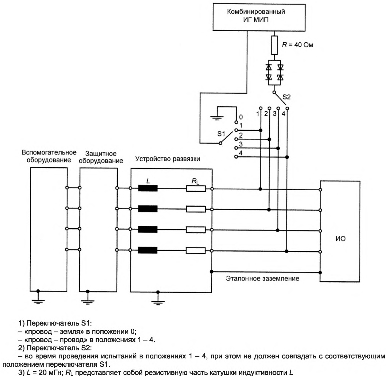
Рисунок 13 – Пример организованного места для испытаний при подаче МИП по схемам «провод – провод» и «провод – земля» с использованием связи через фиксирующую схему на неэкранированные несимметричные линии (в соответствии с 7.3)
