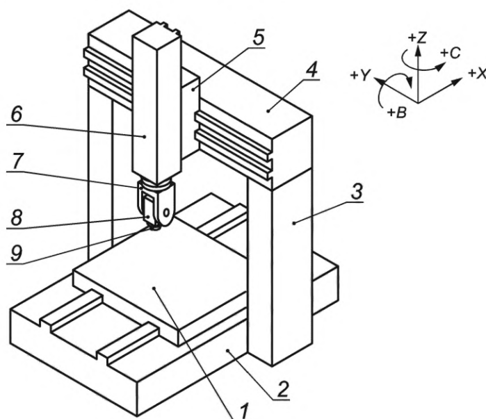
1 — стол (ось X' ); 2 — станина; 3 — стойка; 4 — поперечная балка; 5 — суппорт вертикальных салазок (ось Y ); 6 — вертикальные салазки (ось Z ); 7 — качающаяся головка (ось C ); 8 — наклонная головка (ось B ); 9 — шпиндель [ось (C1) ]
