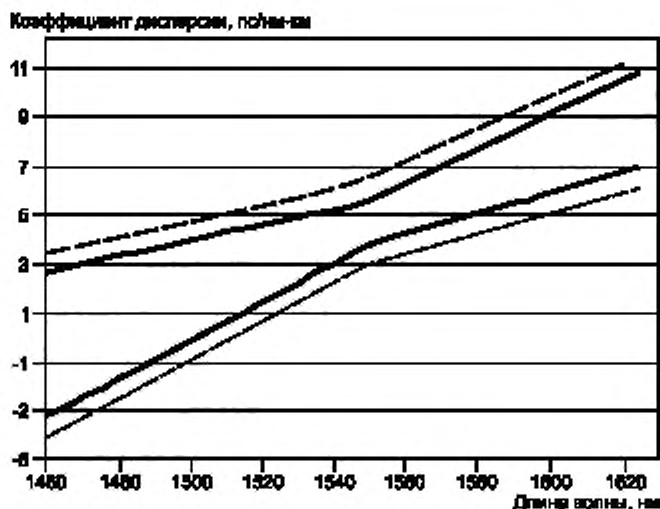
Рисунок Н.1 — Предельные значения коэффициента хроматической дисперсии для ОВ подкатегории B4_d
