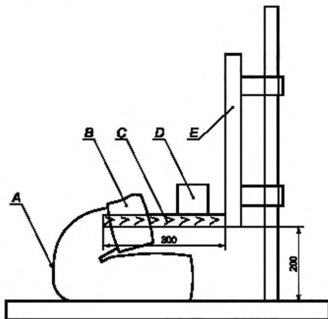
А — грелка для ног; В — отделение для ног; С — доска из фанеры, ширина 150 мм; D — груз; E — подвижная опора
