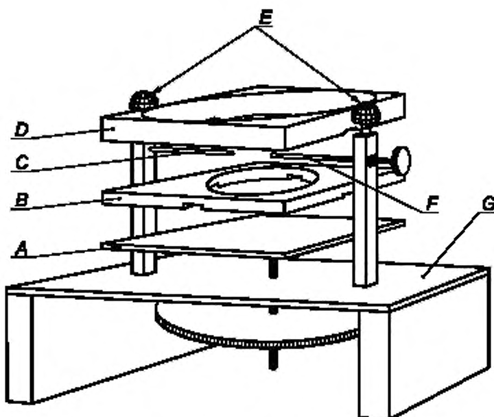
A — регулируемая платформа; B — нижняя часть щита (см. деталь A на рисунке 104); C — неподвижный электрод; D — верхняя часть щита (см. деталь B на рисунке 104); E — зажимы; F — подвижный электрод; G — основная плита
