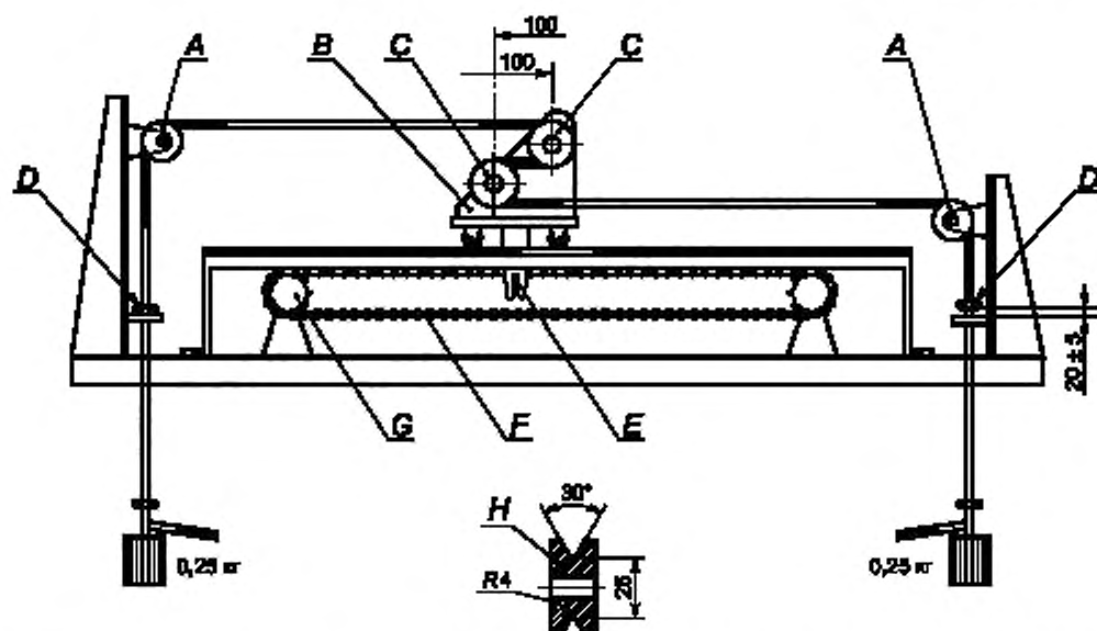
A — шкив диаметром > 50 мм; B — тележка; C — шкив с желобком; D — удерживающий зажим; E — сцепляющий штырь; F — цепь с шагом 12,7 мм; G — цепное колесо с 20 зубцами диаметром начальной окружности 88,9 мм H — подробно о шкиве C
