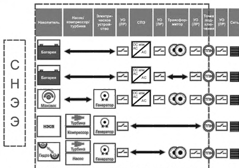
Рисунок 6 — Примеры различных архитектур СНЭЭ
