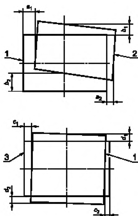
1 — РАДИАЦИОННОЕ ПОЛЕ; 2 — СВЕТОВОЕ ПОЛЕ; 3 — ПОВЕРХНОСТЬ ПРИЕМНИКА ИЗОБРАЖЕНИЯ
