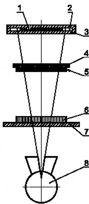
1 — ПОВЕРХНОСТЬ ПРИЕМНИКА ИЗОБРАЖЕНИЯ; 2 — кассета P; 3 — ПРИЕМНИК РЕНТГЕНОВСКОГО ИЗОБРАЖЕНИЯ; 4 — кассета Q; 5 — ТЕСТ-ОБЪЕКТ для проверки ориентирования; 6 — ФАНТОМ для ОСЛАБЛЕНИЯ; 7 — СТОЛ для ПАЦИЕНТА; 8 — БЛОК ИСТОЧНИКА РЕНТГЕНОВСКОГО ИЗЛУЧЕНИЯ
