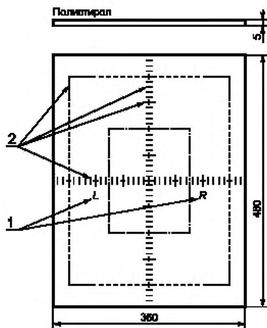
Рисунок 3 — ТЕСТ-ОБЪЕКТ для проверки ориентирования
