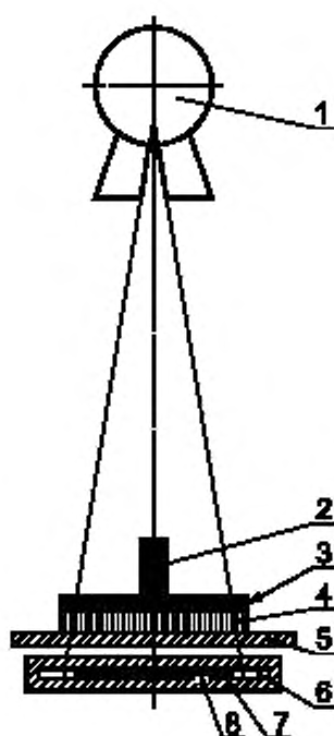
1 — БЛОК ИСТОЧНИКА РЕНТГЕНОВСКОГО ИЗЛУЧЕНИЯ; 2 — ТЕСТ-ОБЪЕКТ для проверки перпендикулярности; 3 — ТЕСТ-ОБЪЕКТ для проверки ориентирования; 4 — ФАНТОМ для ОСЛАБЛЕНИЯ; 5 — КАССЕТА P; 6 — СТОЛ ДЛЯ ПАЦИЕНТА; 7 — ПРИЕМНИК РЕНТГЕНОВСКОГО ИЗОБРАЖЕНИЯ; 8 — ПОВЕРХНОСТЬ ПРИЕМНИКА ИЗОБРАЖЕНИЯ
