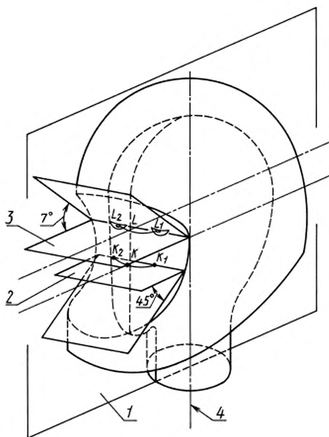
1 — средняя вертикальная плоскость; 2 — основная плоскость; 3 — контрольная плоскость; 4 — центральная вертикальная ось
