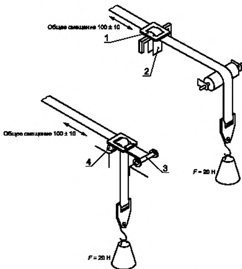
1 — вертикальный и боковой упор; 2 — защитный ремешок, проходящий во внутренней перемычке; 3 — поворотный палец; 4 — нижний стопор
