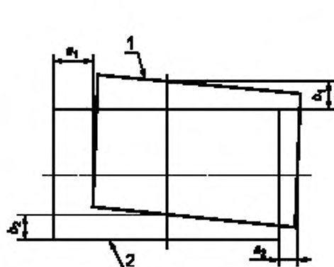
1 — визуально определенное поле; 2 — ПОЛЕ РЕНТГЕНОВСКОГО ИЗЛУЧЕНИЯ
