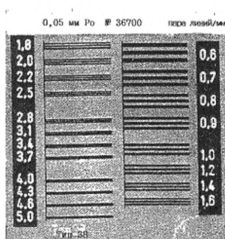
Рисунок 3 — ТЕСТ-ОБЪЕКТ для проверки ПРОСТРАНСТВЕННОГО РАЗРЕШЕНИЯ
