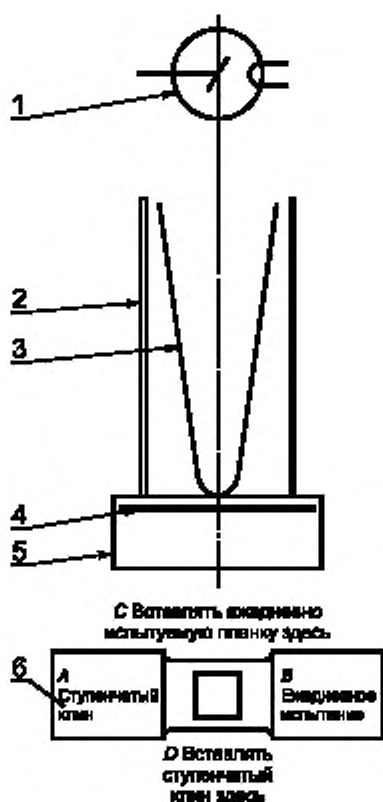
1 — РЕНТГЕНОВСКАЯ ТРУБКА; 2 — цилиндрический тубус; 3 — конический тубус; 4 — фильтр (4,75 мм алюминия); 5 — кожух для закрепления частей А и В ТЕСТ-ОБЪЕКТА; 6 — ТЕСТ-ОБЪЕКТ
