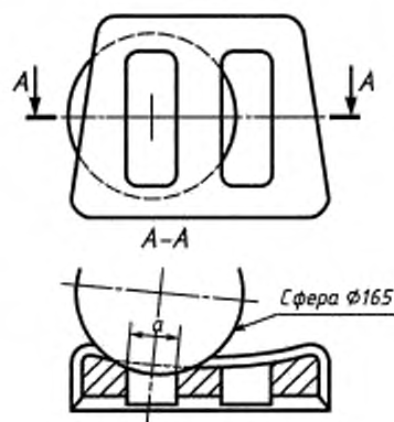
Рисунок 8.2 — Образец вертикального проема
