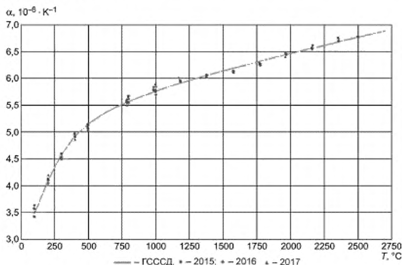
Рисунок А.4 — Сравнение полученных результатов по среднему ТКЛР графита марки ГИП-4 в диапазоне температур от 20 °C до 2500 °C с данными, полученными в 2015—2017 гг. Сплошная линия — значения ССД о ТКЛР графита марки ГИП-4
