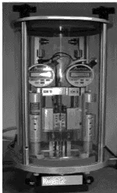
Рисунок А.2 — Конструкция блока индикаторов
