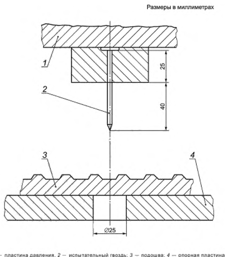
Рисунок 9 — Машина для определения сопротивления проколу подошвы с металлической проколозащитной прокладкой
