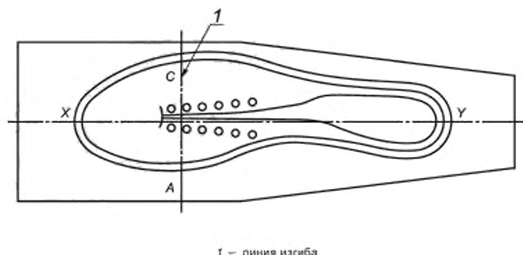
Рисунок 31 — Положение обуви на испытательном аппарате
