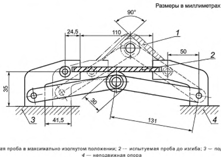
Рисунок 33 — Испытательное устройство для испытания подошвы на изгиб
