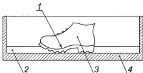
1 — точка измерения температуры; 2 — песчаная баня (высота песка ~ 30 мм); 3 — обувь, заполненная шариками из нержавеющей стали; 4 — нагревательная плита
