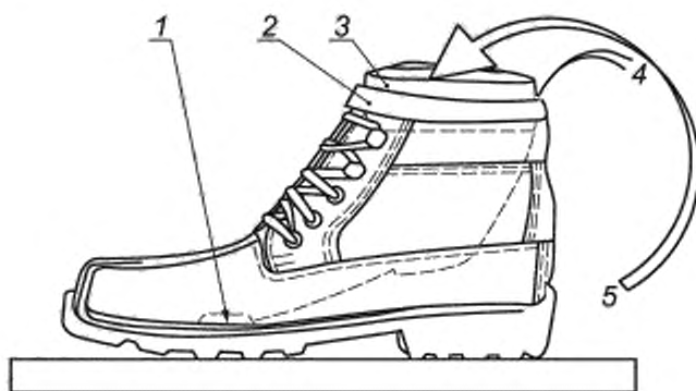
1 — точка измерения температуры; 2 — ленты соединения верха обуви с удлиняющим рукавом; 3 — заглушка; 4 — провода к термодатчику; 5 — стальные шарики (здесь не показаны)
