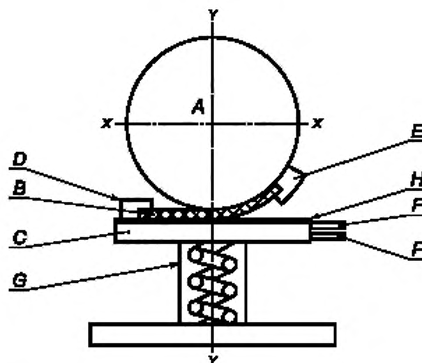
А — медный ролик; В — испытуемая проба; С — платформа; D — зажим на платформе; Е — зажим на медном ролике. F — устройство для подачи воды; G — средство прижима платформы; Н — хлопковая марля
