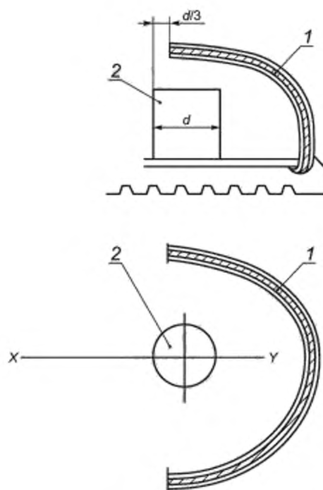
1 — защитный носок, 2 — цилиндр из пластилина; XY — испытательная ось
