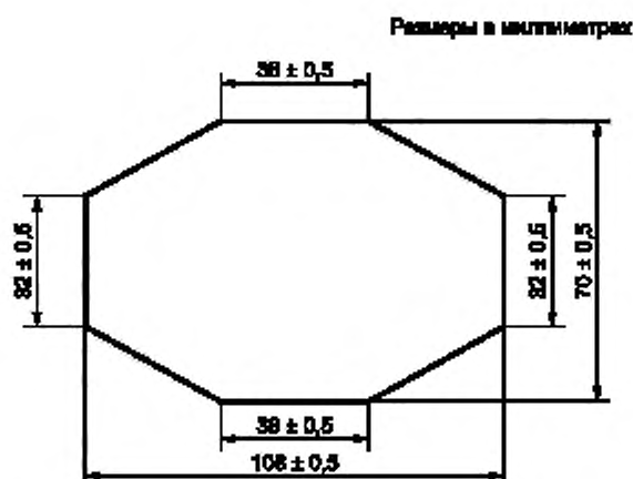
Рисунок 23 — Испытуемая проба для испытания на изгиб
