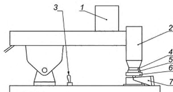
1 — груз; 2 — установленные в корпус нагревательные блоки, включающие устройство измерения температуры; 3 — вкл/выкл тумблер; 4 — квадратный конец медного бита; 5 — испытуемую пробу; 6 — самовыравнивающаяся платформа для испытуемого образца, 7 — шарнирная теплоизолированная опора
