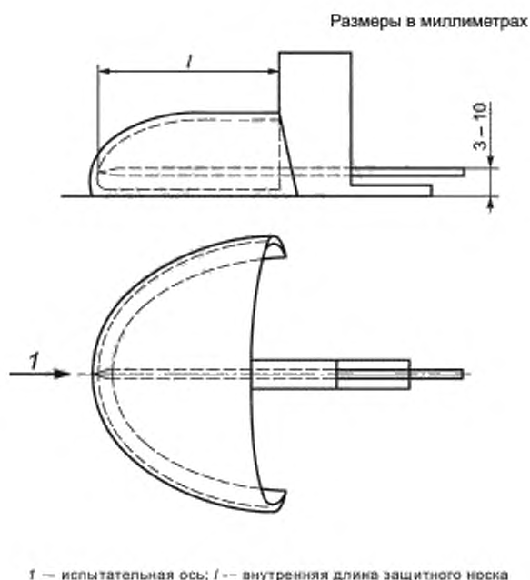
Рисунок 3 — Измерение внутренней длины носка
