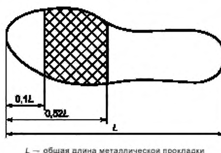
Рисунок 9 — Область проколзащитной прокладки, где не допускается наличие отверстий
