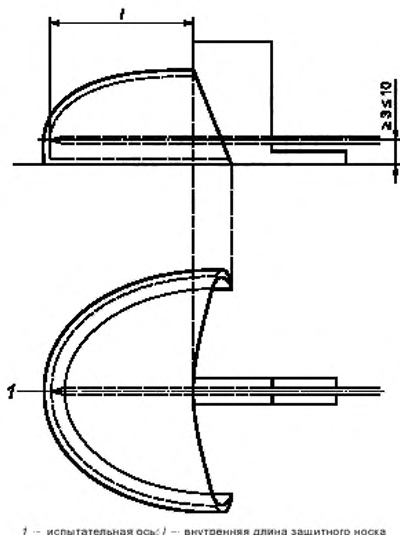
Рисунок 3 — Измерение внутренней длины защитного носка
