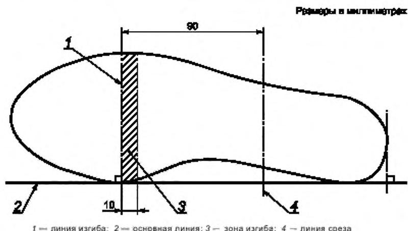
1 — линия изгиба; 2 — основная линия; 3 — зона изгиба; 4 — линия среза
