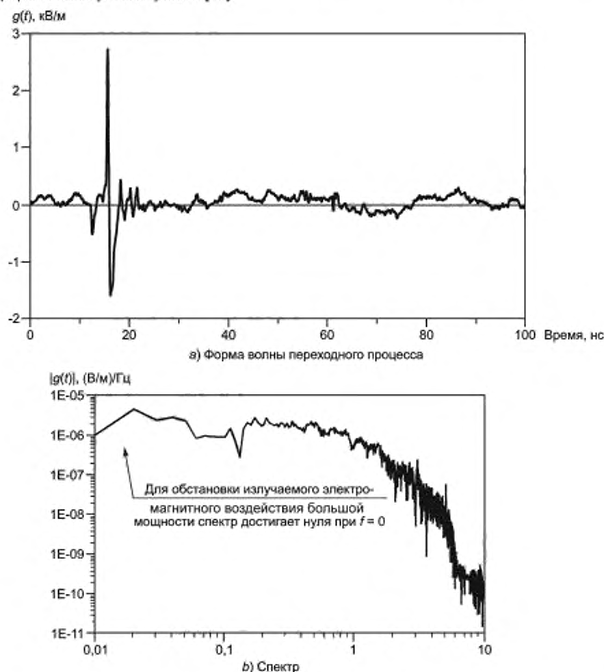
Рисунок 3 — Пример широкополосного переходного процесса электромагнитного воздействия большой мощности вместе с его спектральным представлением
