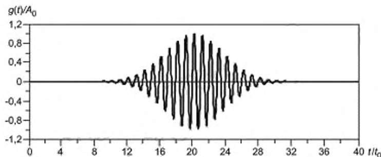
а) Форма волны переходного процесса
