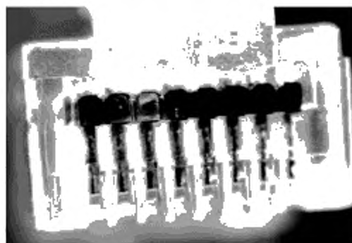
Рисунок 9 — Пример повреждения, вызванного одиночным импульсом «телекоммуникационного» генератора при напряжении 4,5 кВ
