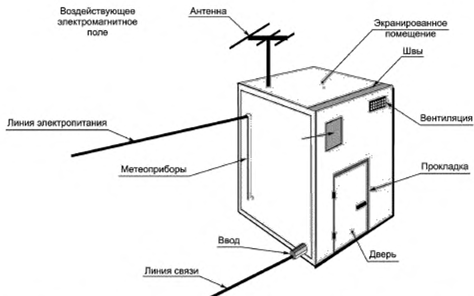
Рисунок 5 — Упрощенная схема гипотетического сооружения, облучаемого внешним электромагнитным полем
