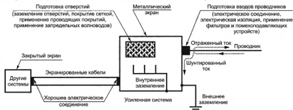
Рисунок 14 — Типичные способы защиты ненамеренно созданных путей электромагнитного проникновения
