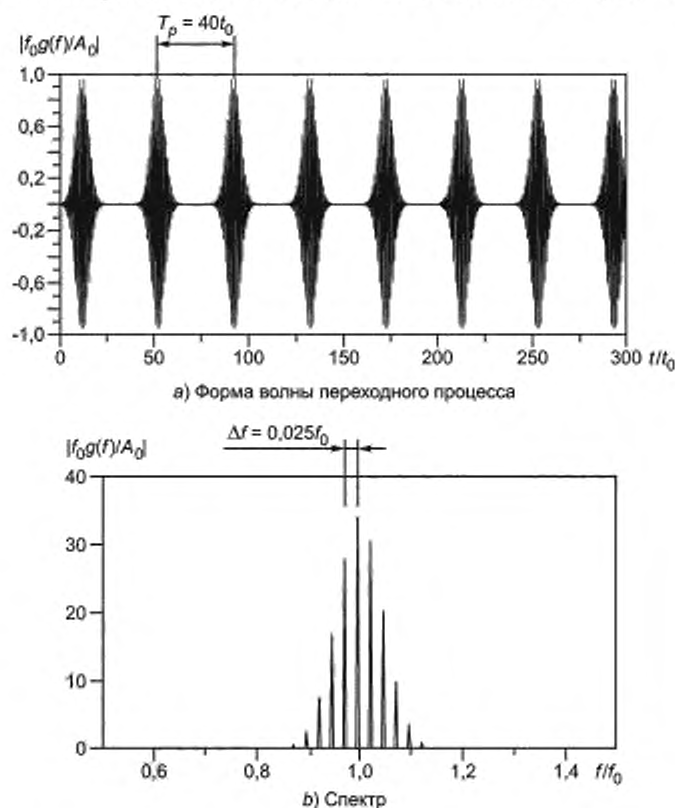
Рисунок 4 — Пример повторяющихся импульсов, аналогичных представленному на рисунке 2
