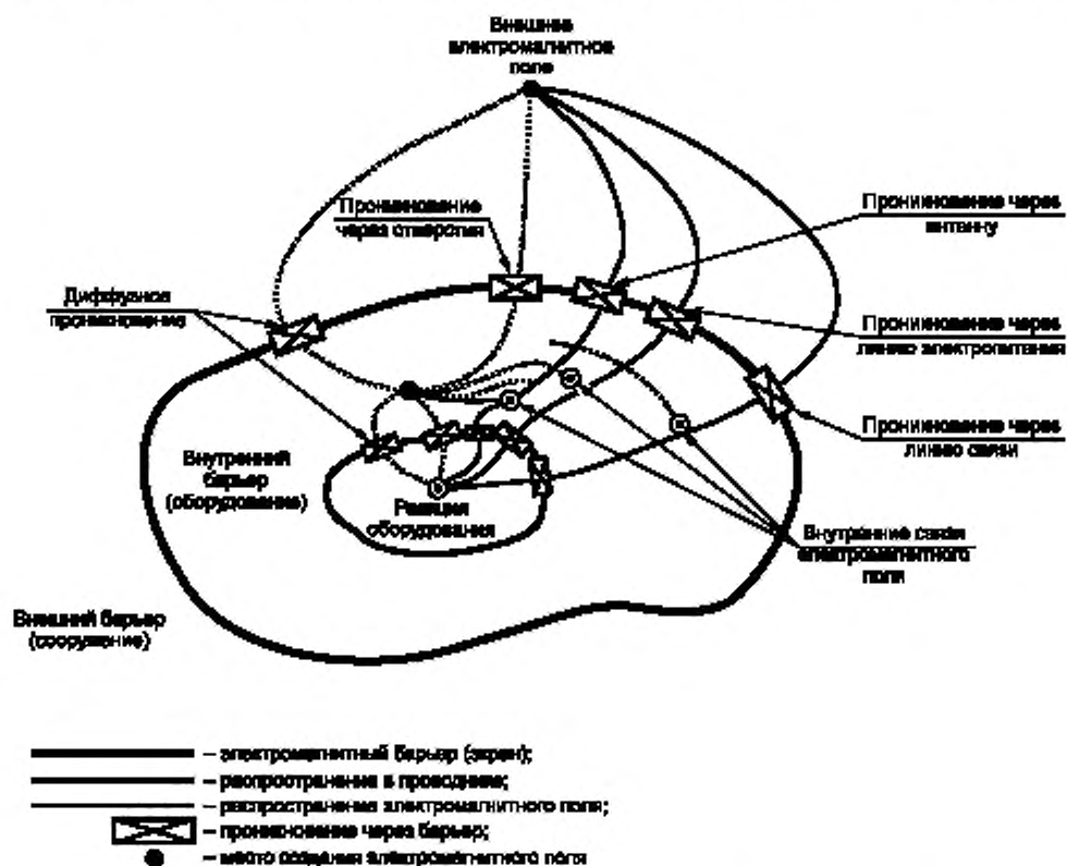
Рисунок 6 — Топологическая схема для простой системы, представленной на рисунке 5
