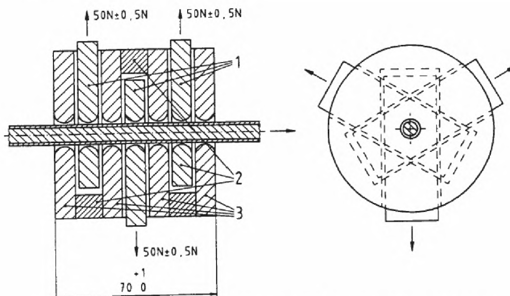
Рисунок 3 – Устройство для испытания на смещение оболочки
