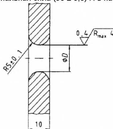
Рисунок 4 – Поперечное сечение отверстий
