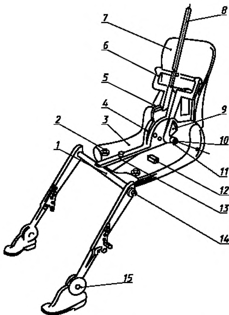
1 — коленный Т-образный шарнир; 2 — кронштейн набедренных грузов; 3 — основание; 4 — круговой сектор наклона бедра; 5 — уровень угла наклона спинки; 6 — кронштейн спинных грузов; 7 — спинка; 8 — штырь; 9 — круговой сектор наклона спинки; 10 — визирные метки точки H ; 11 — ось вращения точки H ; 12 — поперечный уровень; 13 — кронштейн бедра; 14 — круговой сектор сгиба колена, 15 — круговой сектор сгиба ступни
