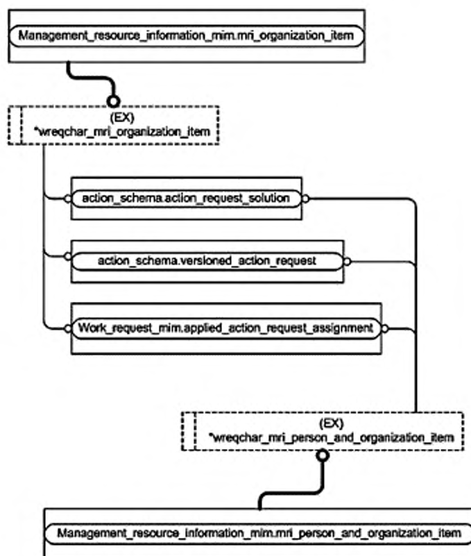
Рисунок D.5 — Представление ИММ на уровне объектов в формате EXPRESS-G. Диаграмма 4 из 5
