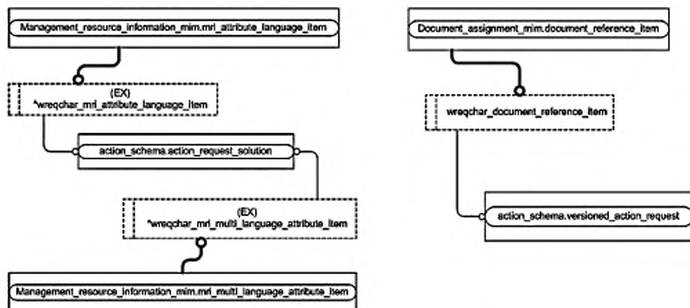
Рисунок D.6 — Представление ИММ на уровне объектов в формате EXPRESS-G. Диаграмма 5 из 5
