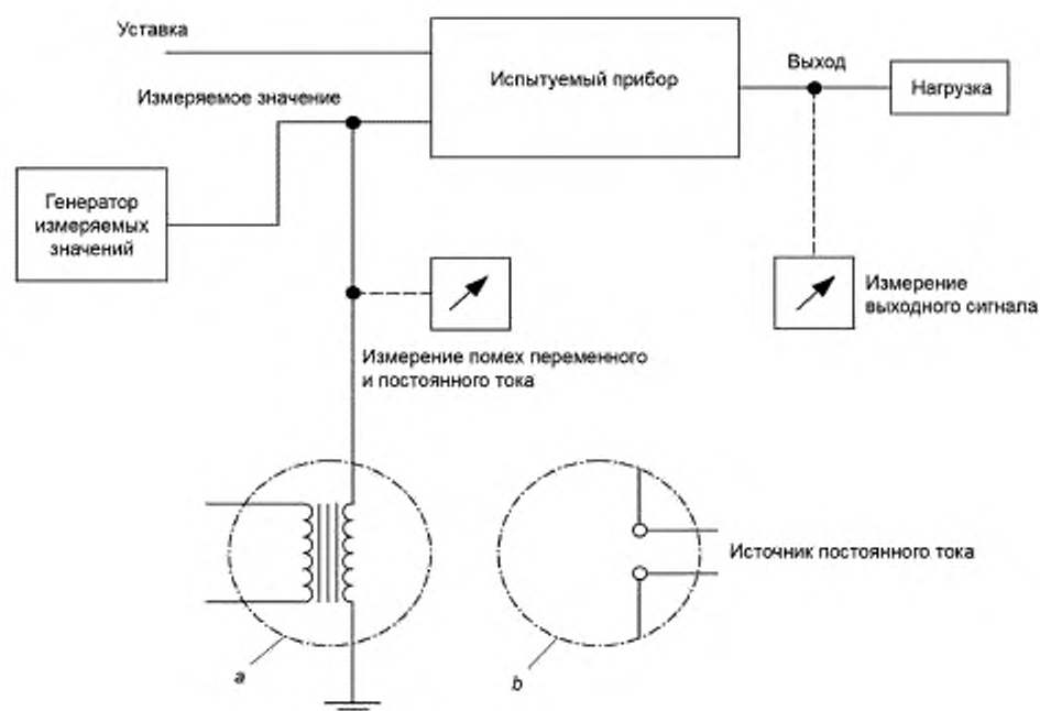
Рисунок 2 — Схема испытания на влияние синфазных помех
