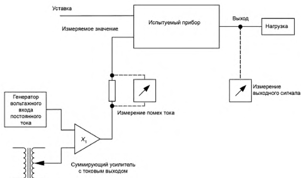
Рисунок 3b — Точковый вход
