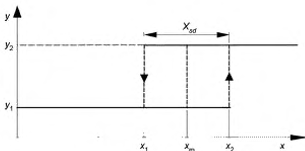
Рисунок 1 — Прибор с двумя устойчивыми состояниями
