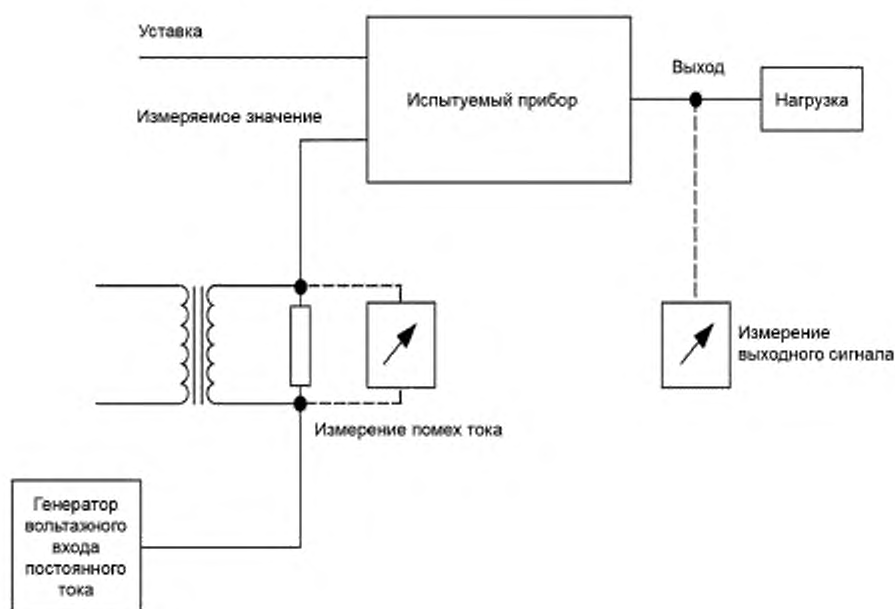
Рисунок 3а — Вольтажный вход
