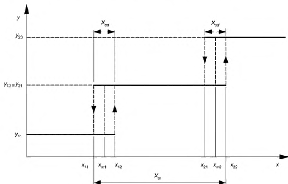
Рисунок 4 — Прибор с тремя устойчивыми состояниями
