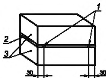
1 — металлические стержни, 2 — мертель, 3 — кирпичи
