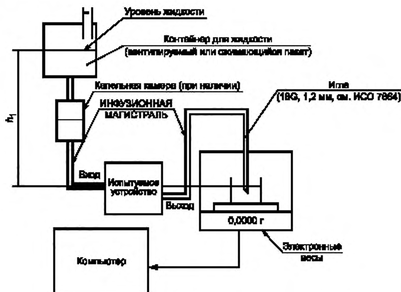
Рисунок 201.104а — Испытательный стенд для ВОЛКУМЕТРИЧЕСКИХ ИНФУЗИОННЫХ НАСОСОВ и для ВОЛКУМЕТРИЧЕСКИХ ИНФУЗИОННЫХ КОНТРОЛЛЕРОВ
