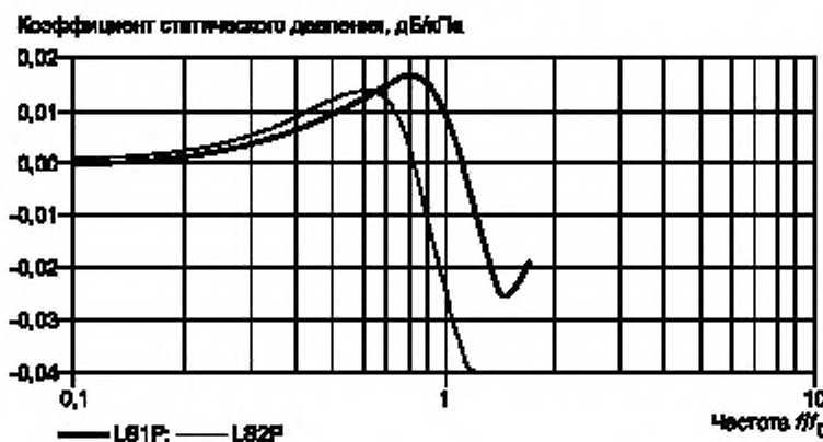
Рисунок Г.1 — Примеры зависимости коэффициентов статического давления для микрофонов типов LS1P и LS2P от относительной частоты f/f_0 .
