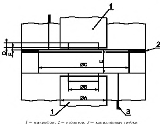
Рисунок В.2 — Эскиз камеры связи большого объема
