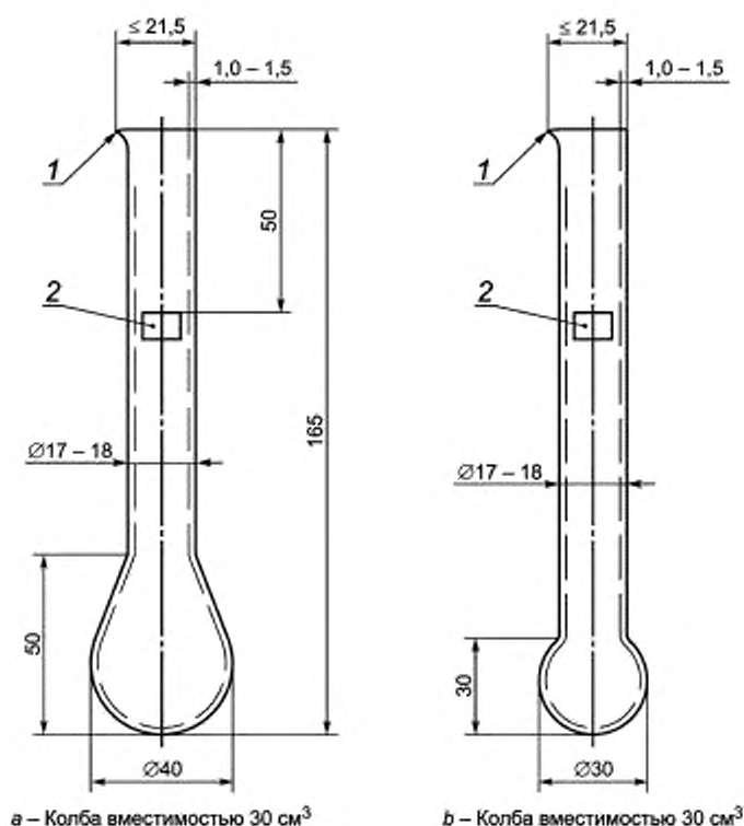
Рисунок 2 — Выпускная трубка для полумикрометода
