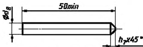
Рисунок 105 — Калибр для проверки фазных гнезд
