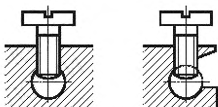
Рисунок IV.1b — Выводы без прижимных пластин
