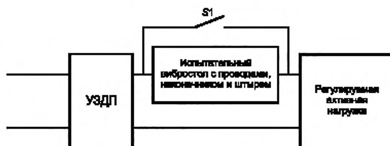
Рисунок F.3 — Соединение УЗД с вибростолом при испытании
