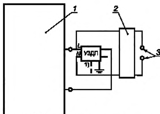
1 — генератор импульсного тока 8/20 мкс; 2 — фильтр; 3 — источник питания
