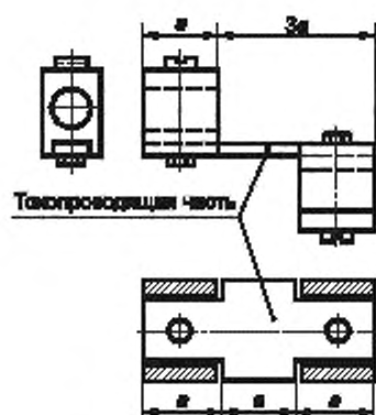
Рисунок L.6 — Пример присоединения выводов УЗДП
