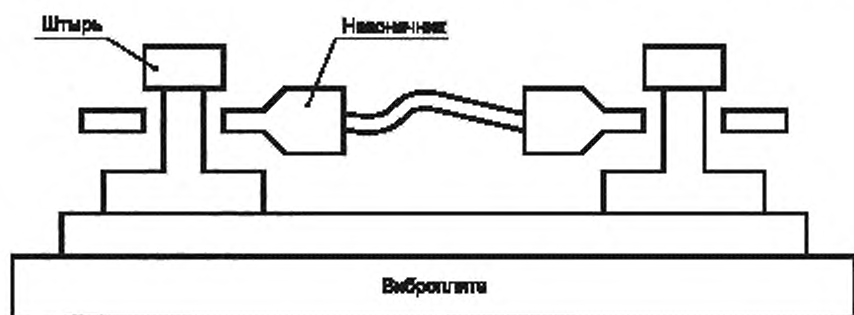
Рисунок F.2 — Испытательный вибродоменный стол для дуговых испытаний ослабленных зажимов
