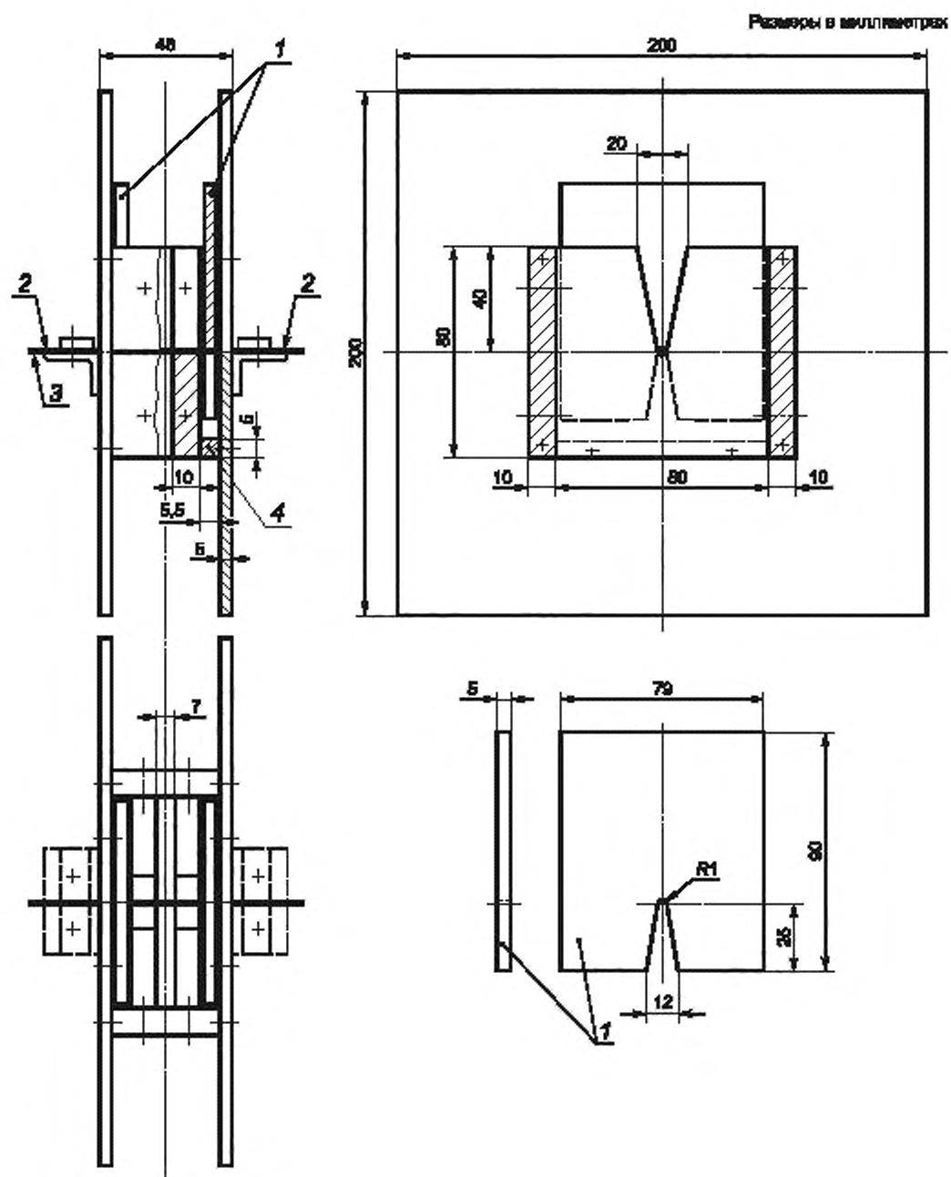
Рисунок IE.1 — Испытательное устройство для проверки устойчивости УЗДП к минимальным значениям R_{ti} и I_p
