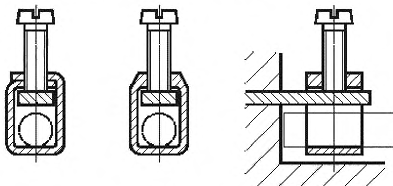
Рисунок IV.1a — Выводы с хомутиком
