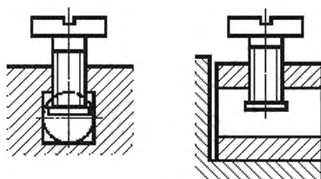
Рисунок IV.1c — Выводы с прижимными пластинами
