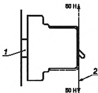
1 — рейка; 2 — шнур
