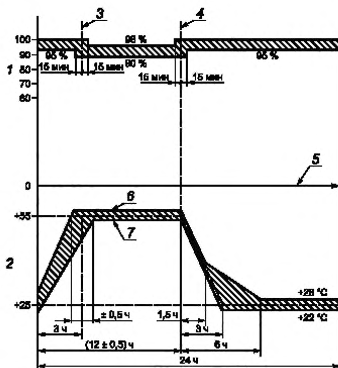
1 — относительная влажность, %; 2 — температура окружающей среды, °C; 3 — окончание повышения температуры; 4 — начало падения температуры; 5 — время; 6 — верхняя предельная температура 57 °C; 7 — нижняя предельная температура 53 °C
