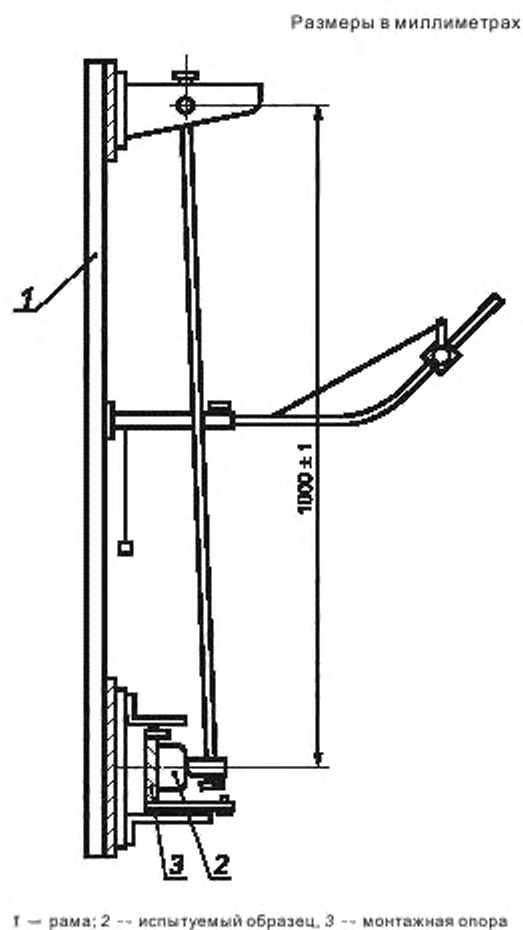
Рисунок 24 — Устройство для испытания на механический удар (9.12.2.2)
