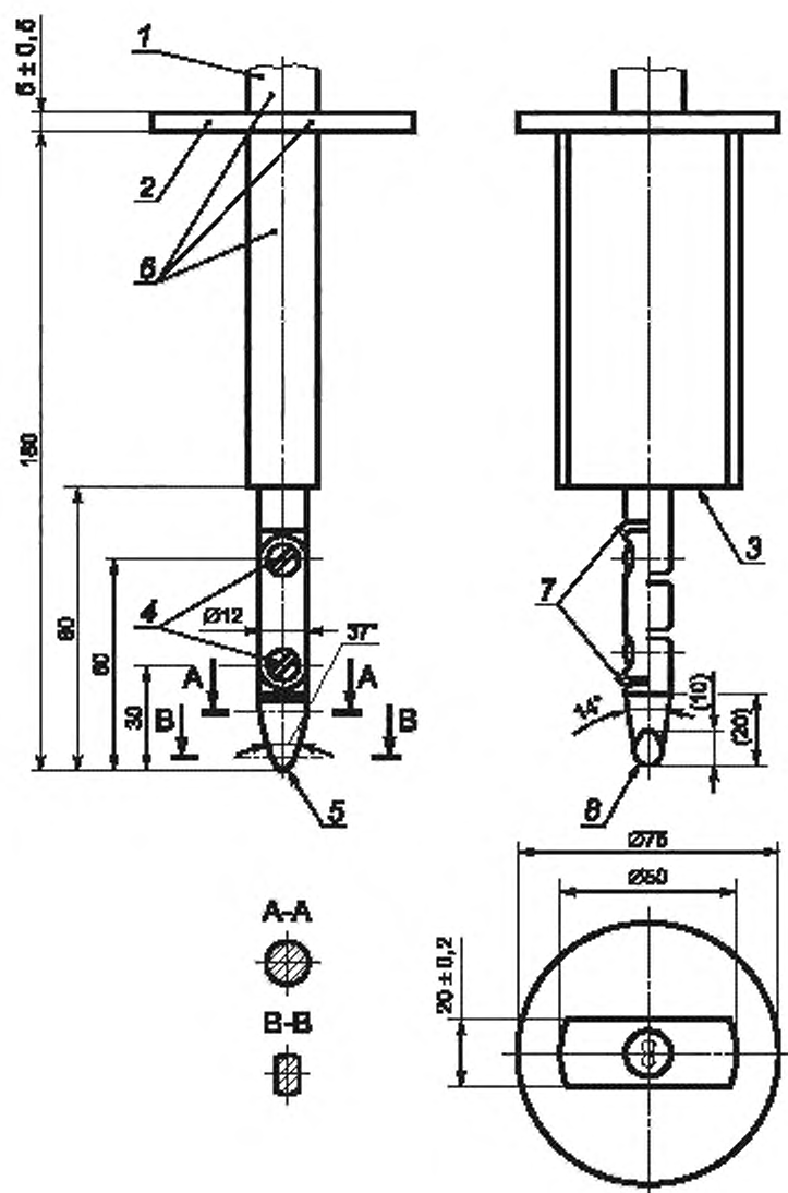
1 — рукоятка; 2 — ограждение; 3 — упор; 4 — шарниры; 5 — скругление R2 \pm 0,05 ; 6 — изоляционный материал; 7 — притупленные кромки; 8 — скругление R4 \pm 0,05
