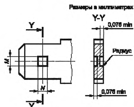
Рисунок К.4 — Размеры прямоугольных углублений фиксации (см. рисунок К.2)
