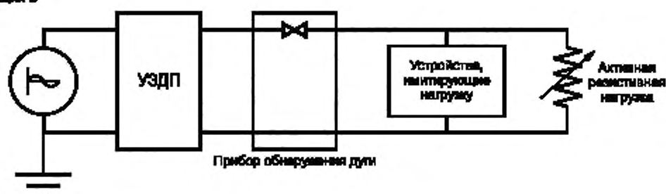
Рисунок 11 — Конфигурации цепей испытания устойчивости к фоновым помехам
