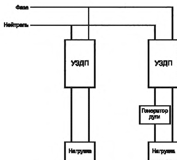
Рисунок 16 — Цепь для испытания при перекрестных помехах
