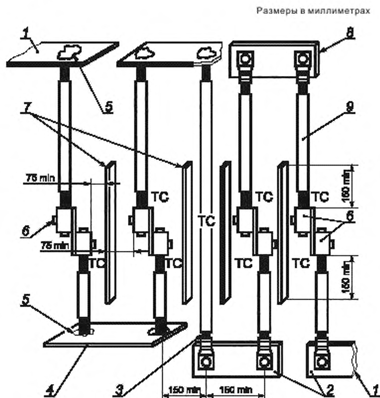
1 — подвод питания; 2 — эквалайзеры; 3 — контрольный проводник; 4 — шина эквалайзера; 5 — сварка; 6 — испытуемый образец; 7 — термоизолирующая перегородка (4 шт.); 8 — шина; 9 — испытательный проводник; TC — термopapa
