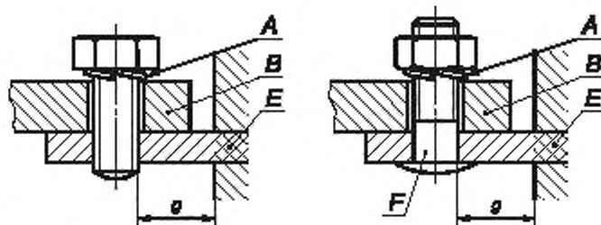
A — запорное устройство; B — кабельный наконечник или шина; E — неподвижная часть, F — штырь
