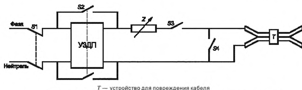
Рисунок 7 — Цель для испытания на параллельный дуговой пробой при повреждении кабеля
