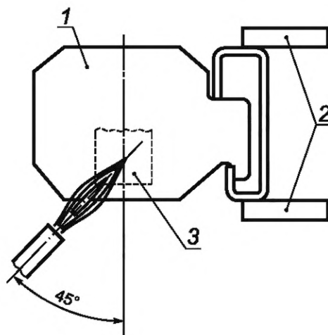
1 — клеммная колодка; 2 — фиксирующие части; 3 — часть колодки в области выводного зажима
