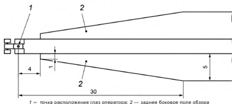
Рисунок 1 — Заднее боковое поле обзора
