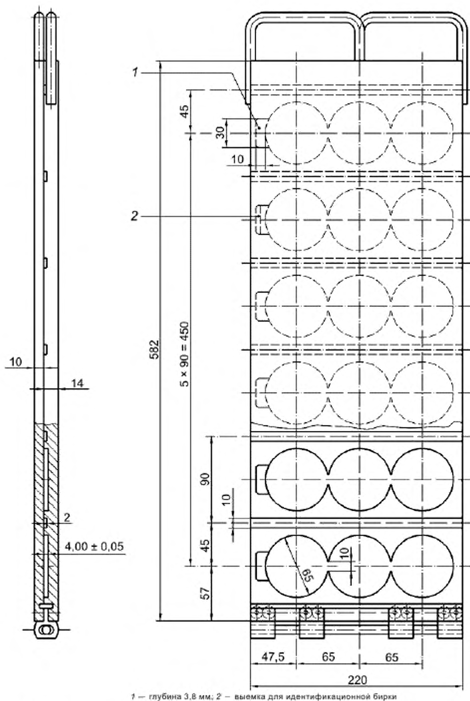
Рисунок 2 — Пресс-форма для вулканизации дисков для получения образцов в форме колец
