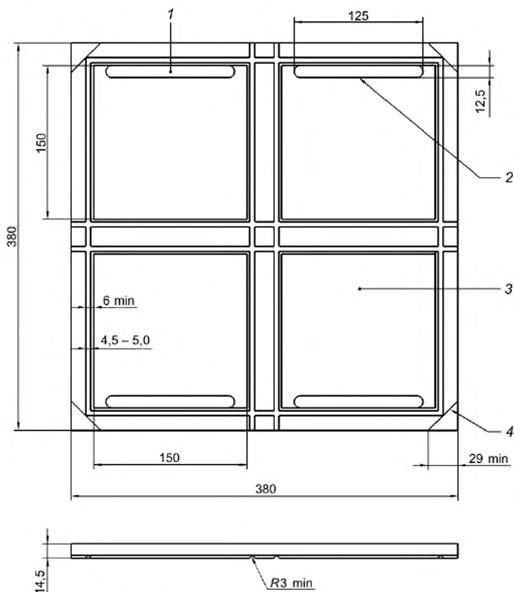
Рисунок 1 — Четырехгнездная пресс-форма
