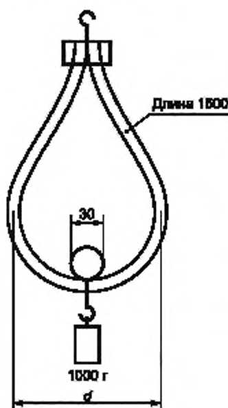
Рисунок 16 — Подготовка шлангов для испытания на гибкость
