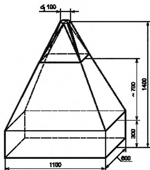
Рисунок 25 — Испытательный кожух
