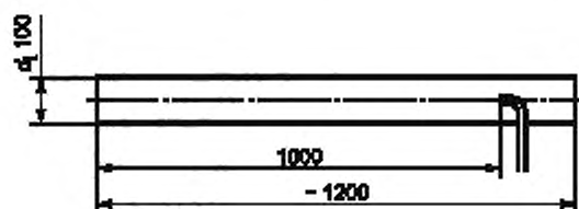
Рисунок 27 — Выхлопной канал с выборкой для исследования
