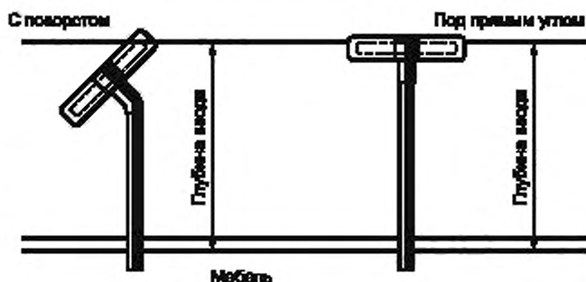
Рисунок 12 — Глубина ввода
