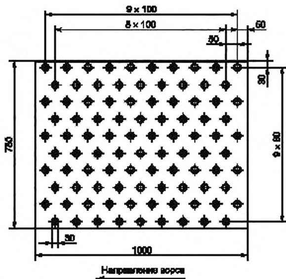
Рисунок 3 — Трафарет для распределения волокон по испытательным коврам
