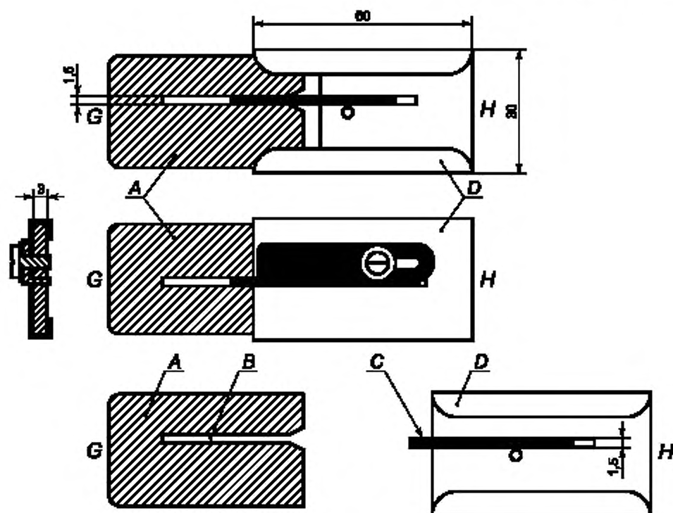
A — стальная пластина; B — прорезь; C — стальной язычок; D — направляющие
