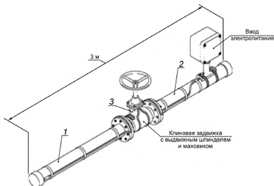
Рисунок 14 — Температурное испытание sprinkлерной системы с ответвлением. Альтернативная обвязка пне,с
